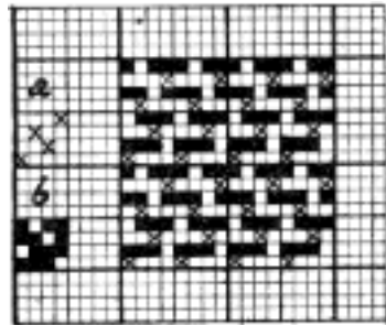
Č. 4323. Vazba pro tkaninu dvojútkovou. a vazba útku vrchního, b vazba útku zpodního.
