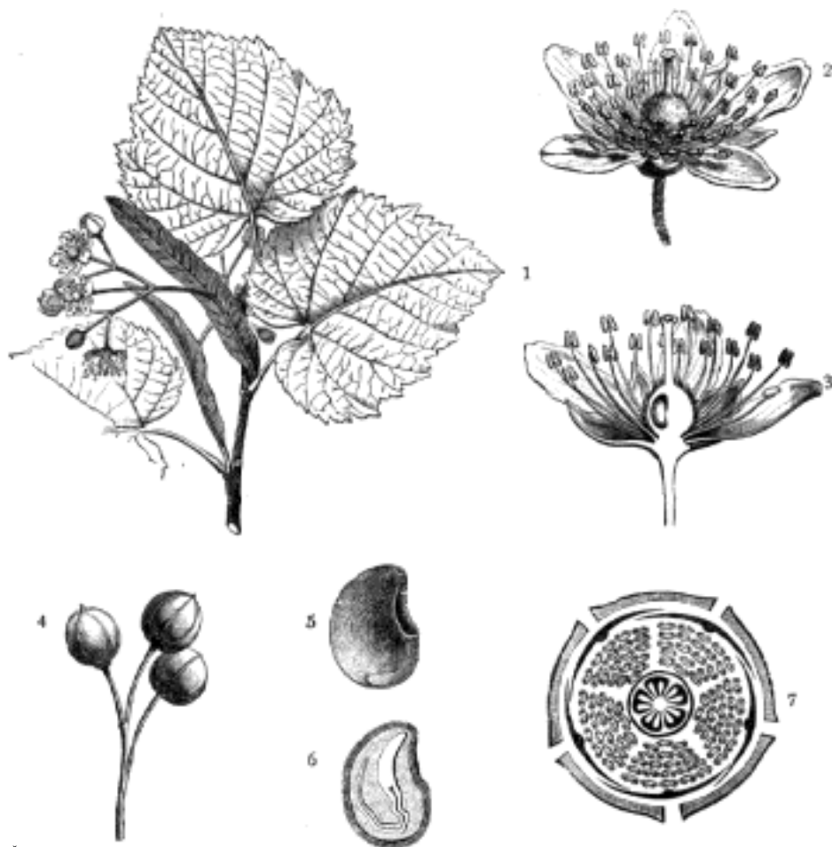
Č. 4308. Tilia : 1. Větvička s květy. - 2. Jednotlivý květ a 3. jeho průřez podélný. - 4. Plody. - 5. Semeno a 6. jeho podélný průřez. - 7. Diagramm květu.
