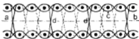
Č. 4329. Dvojný aksamit, a b řez nože, c osnova základní, d osnova vlasová.
