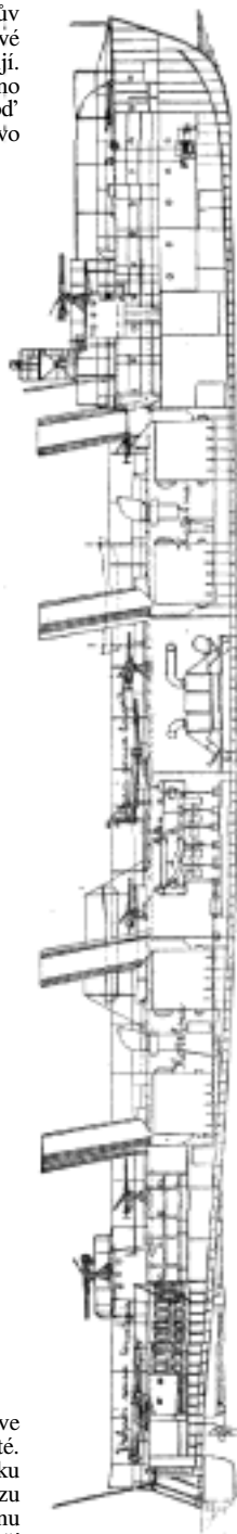
Č. 4369. Řez torpédoborcem.
