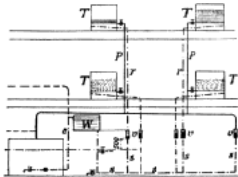
Č. 4351. Topení parou o nízkém tlaku soustavy Körtingovy.
