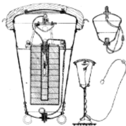
Č. 4364. Vnitřní úprava miny.
