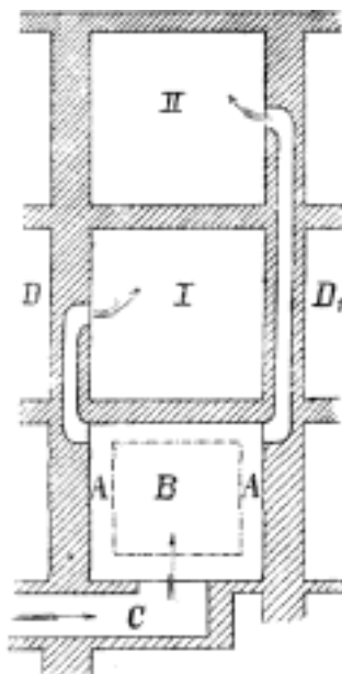
Č. 4342. Topení teplým vzduchem.
