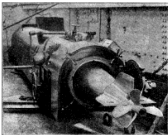
Č. 4366. Roura lancirovací.
