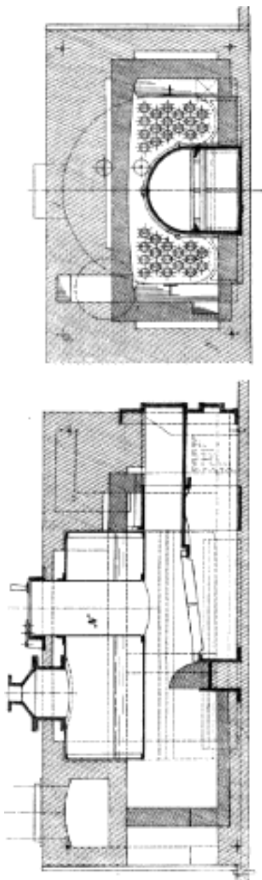
Č. 4345. Kotel k parnímu topení o nízkém tlaku.
