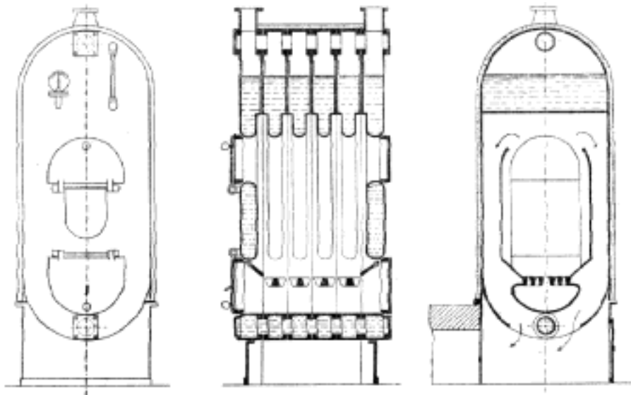
Č. 4346. Kotel s litinovými články.
