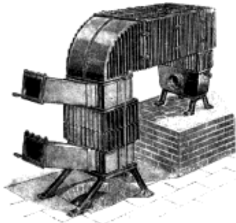
Č. 4343. Kolorifer.
