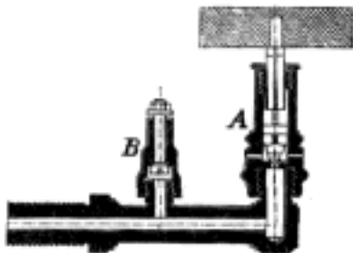
Č. 4357. Expandní armatura při topení teplou vodou.
