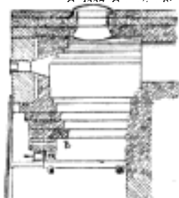
Č. 4338. a 4339. Příčný a podélný řez generátorem.
