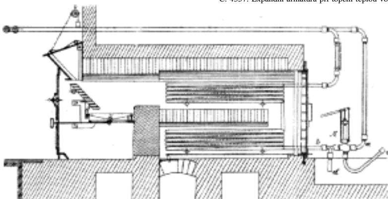
Č. 4357. Expandní armatura při topení teplou vodou.
