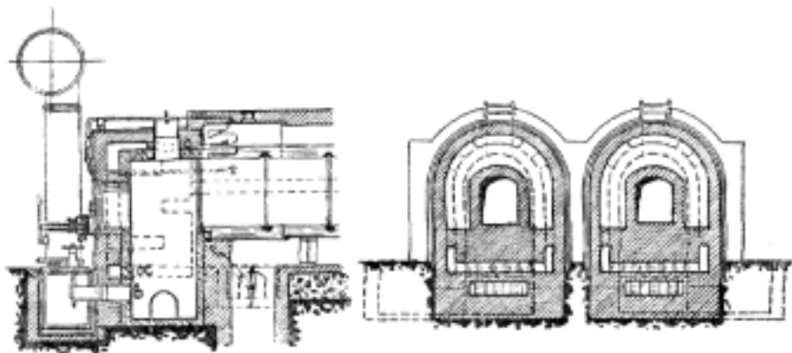
Č. 4341. Topení na spalování plynů kychtových při plamencových kotlích závodů Schneiderových v Creuzotu.
