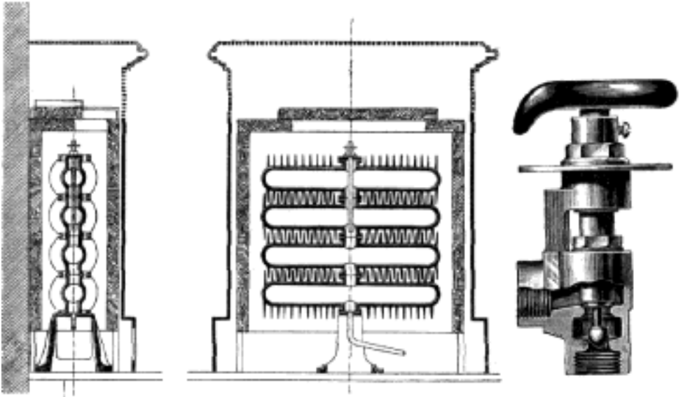
Č. 4352. Topná tělesa o žebrovém povrchu s izolačním pláštěm. Č. 4354. Regulační ventil.
