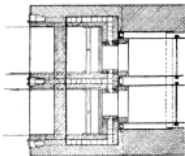
Č. 4336. Topení poloplynové, předkotelní s roštěm stupňovým při kotlu plamencovém.
