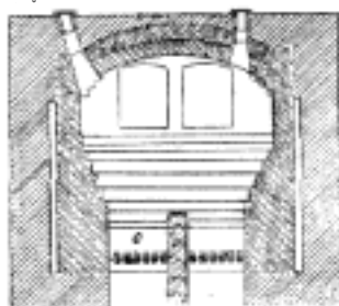
Č. 4338. a 4339. Příčný a podélný řez generátorem.
