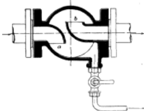
Č. 4355. Odvodňovací vložka k parnímu potrubí.
