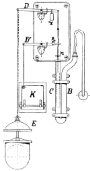
Č. 4348. Rtuťový regulátor.
