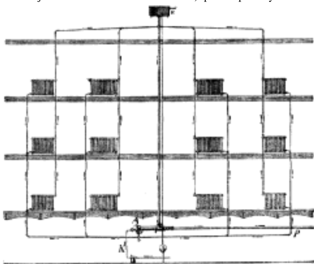
Č. 4360. Topení teplou vodou, zahřívání parou.
