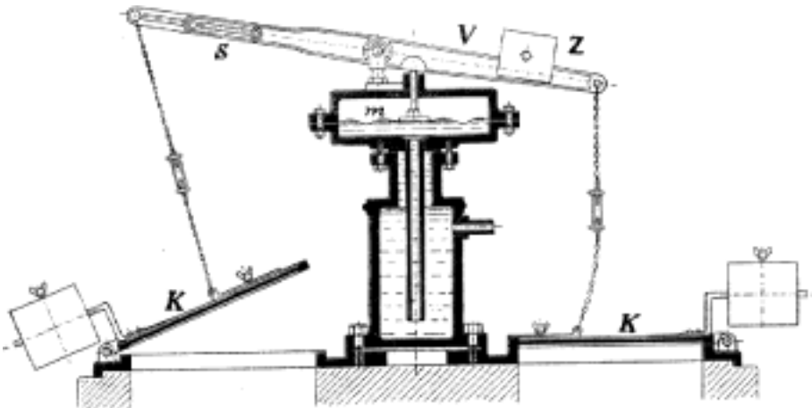
Č. 4349. Membránový regulátor.
