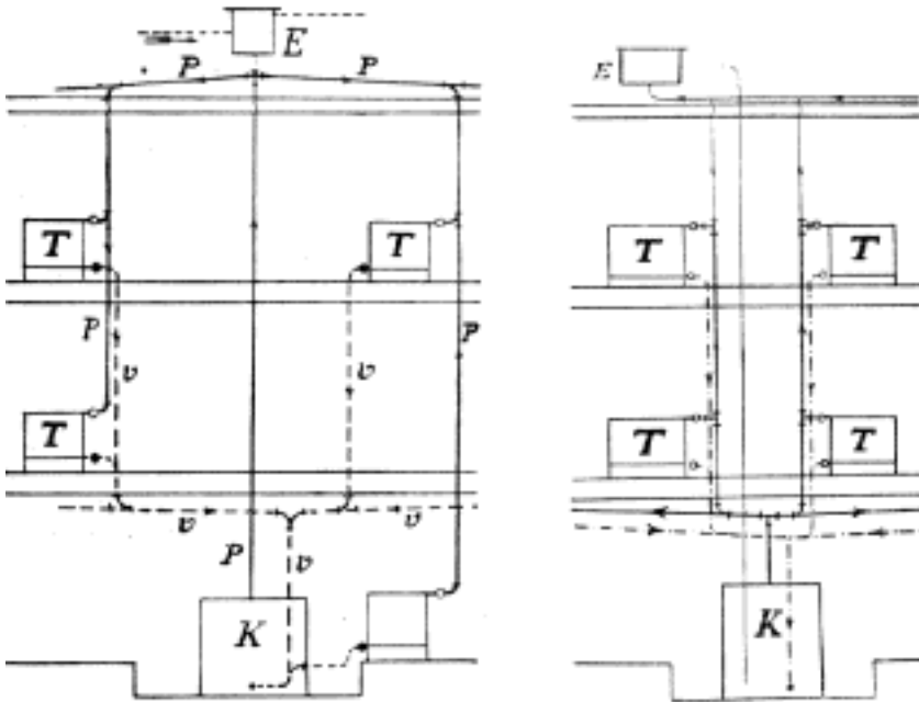
Č. 4358. Topení teplou vodou svrchním rozvodem. Č. 4359. Topení teplou vodou rozvodem spodním.
