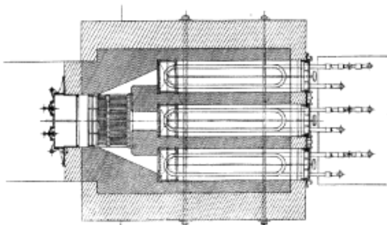
Č. 4356. Vyvíječ tepla k topení teplou vodou.
