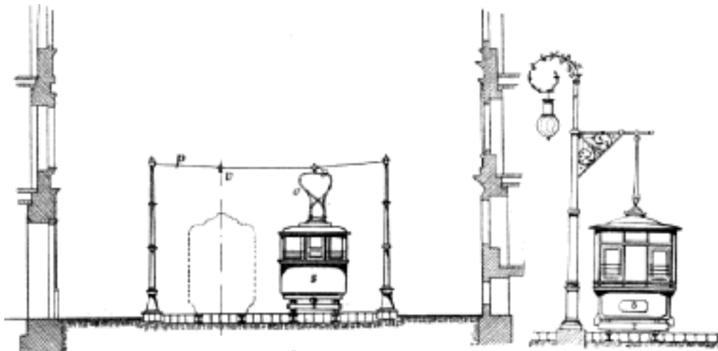
Č. 4381. Upevnění drátů příčných na stožárech. Č. 4382. Ozdobný sloup s jedním příčným rmenem k upevnění drátu jízdního.
