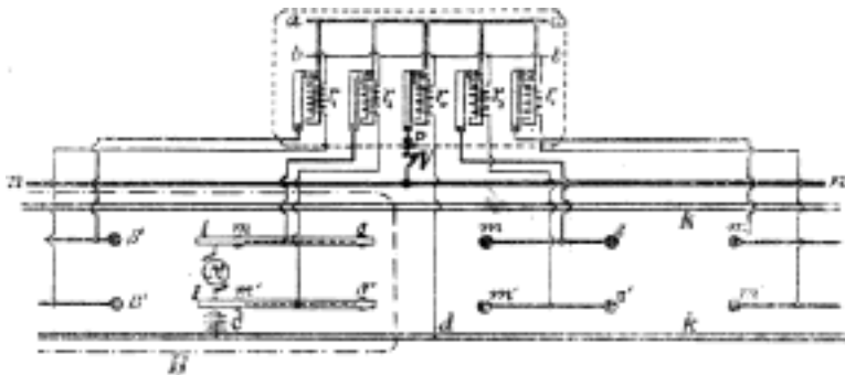
Č. 4387. Rozvod proudový u elektr. tramwaye na mostě Karla IV. v Praze.
