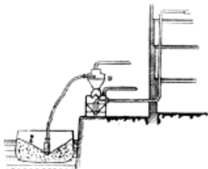
Č. 4401. Vzduchový transporteur pobřežní.
