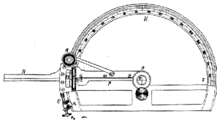
Č. 4405. Noniový transporteur s ustanovkou.
