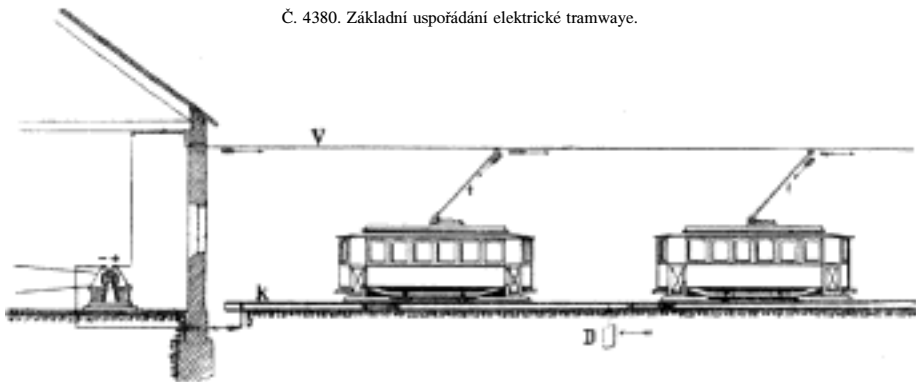
Č. 4380. Základní uspořádání elektrické tramwaye.
