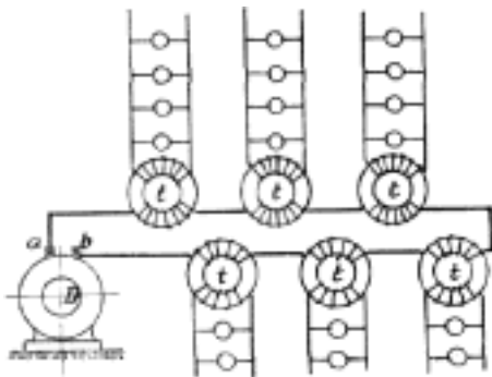
Č. 4397. Sériové spojení transformátorů.
