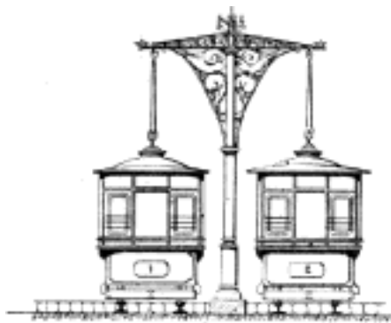
Č. 4383. Ozdobný sloup s dvěma rameny příčnými k upevnění jízdního drátu.
