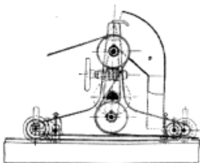
Č. 4400. Transporteur pásový »výpad«.
