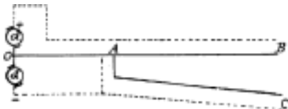
Č. 4386. Tramwayová síť třívodičová.
