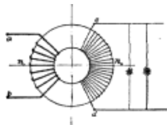
Č. 4394. Princip transformátoru.
