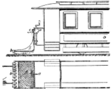
Č. 4389. Síť ochranná s kladkami.
