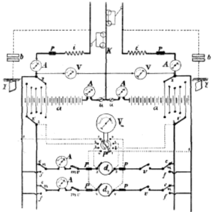
Č. 4385. Centrála třívodičová.
