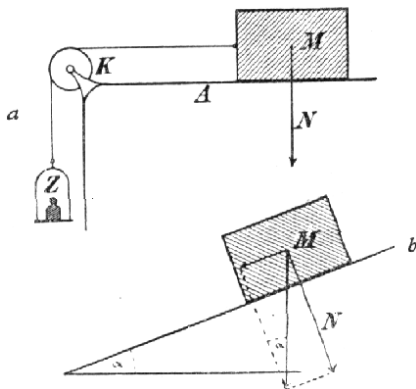
Č. 4413. Tření vlačné.
