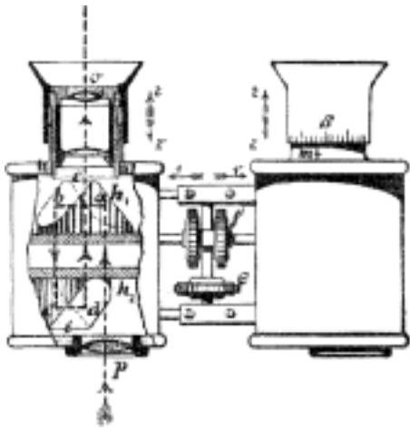
Č. 4415. Triéder-binoce.
