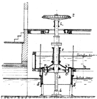
Č. 4451. Řez turbínou Henschel-Jonvalovou.
