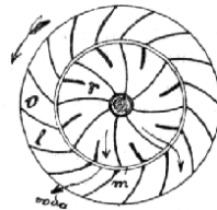
Č. 4450a. Půdorys lopatkových kol turb. Fourneyronovy.
