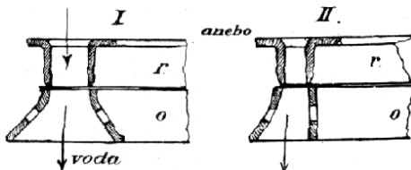
Č. 4447. Střední řez turbinou Girardovou.
