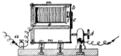
Č. 4439. Občejná trubka elektrická.
