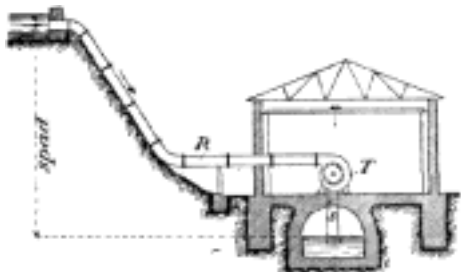
Č. 4460. Dispozice turbíny spirální.
