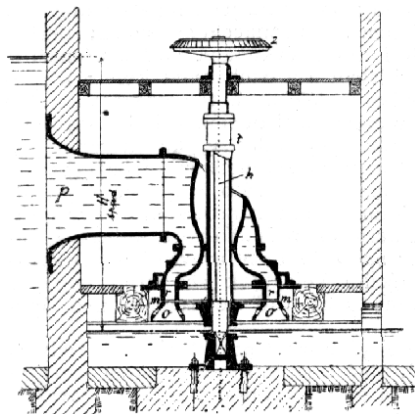
Č. 4452. Řez turbínou Girardovou.
