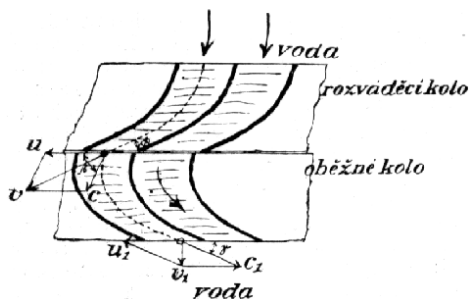
Č. 4446. Rozvinutý střední řez turbinovými věnci.
