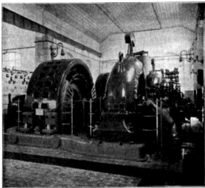
Č. 4459. Francisova turbína spirální pro pohon generátoru elektrického.
