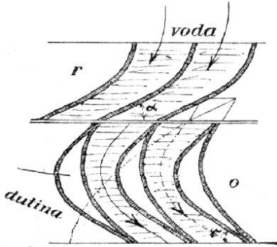
Č. 4449. Rozvinutý řez turbínou s Hänelovými lopatkami.
