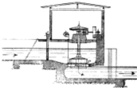
Č. 4456. Turbína Francisova.
