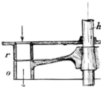
Č. 4448. Střední řez koly turbíny reakční.
