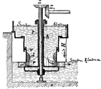
Č. 4450. Řez turbínou Fourneyronovou.
