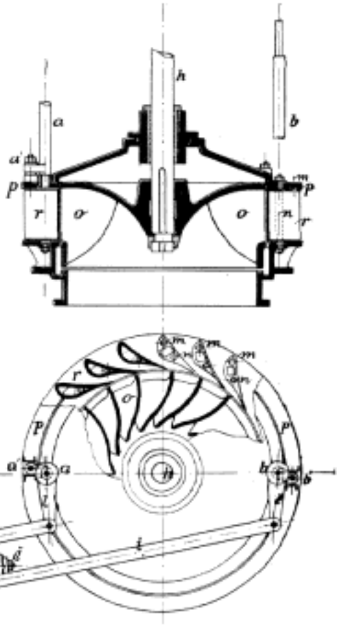
Č. 4457. Turbína Francisova v řezu s regulací.
