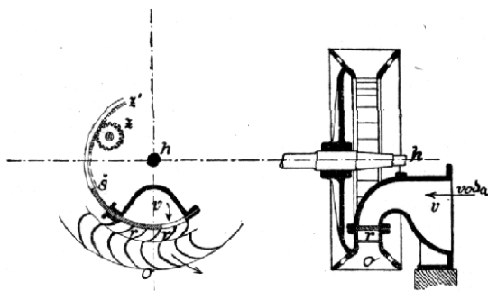
Č. 4453. Turbína Schwamkrugova.
