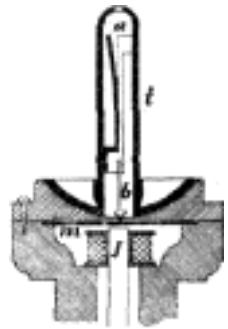
Č. 4438. Telefonní trubka elektrická.
