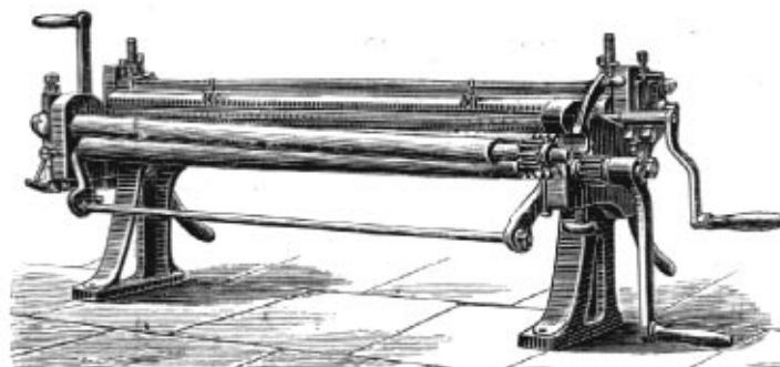
7. a 8. Ohraňovadlo kombinované s ohybačkou, zakružením a podvalovačkou.
