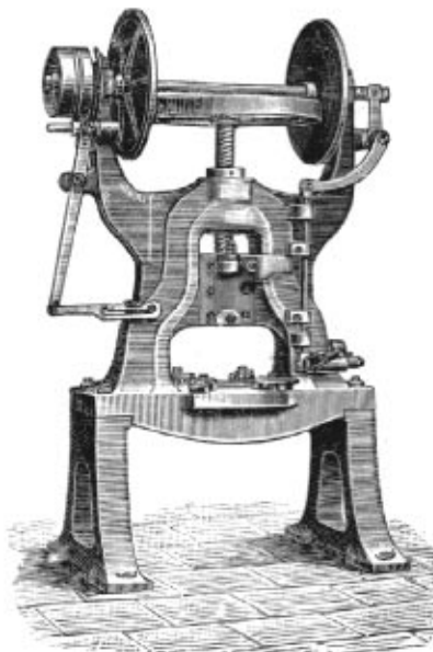
4. Razidlo šroubové s třecími koly.
