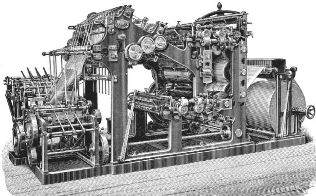
Rotační stroj pro tisk novin.
