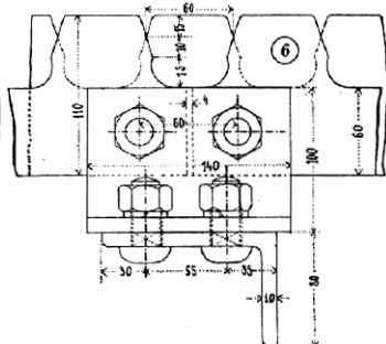
Noty o železných prazích přičných na lanové dráze Litenky v Itale 5-6
