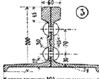
Soustava dvojdielná Hlaarmannova
