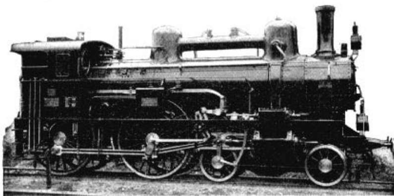
Lokomotiva rychlíková se sdruženým parním strojem c. k. rak. stát. drah (váha vystr. 55.7 t).
