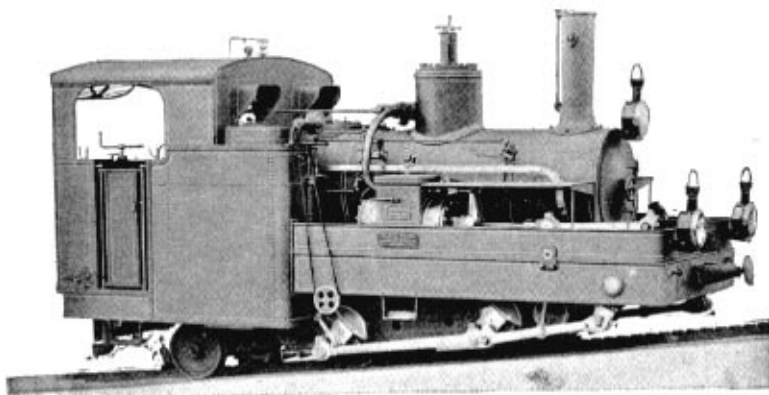
Lokomotiva ozubnicová system Abt pro dráhu Monte-Generoso (váha vystr. 17 t).
