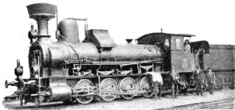
Lokomotiva nákladní čtyřosá c. k. rak. stát. drah (váha vystr. 55 t).
