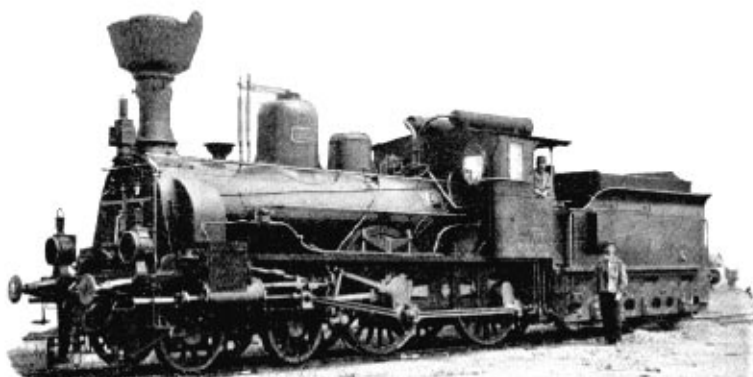
Lokomotiv osobní c. k. rak. stát. drah s tendrem (váha vystr. 45.1 t).
