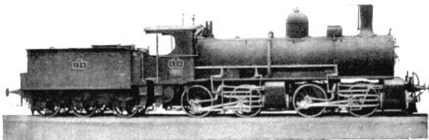
Malletova lokomotiva sdružená pro švýcar. dráhu centrální (váha vystr. 57 t).
