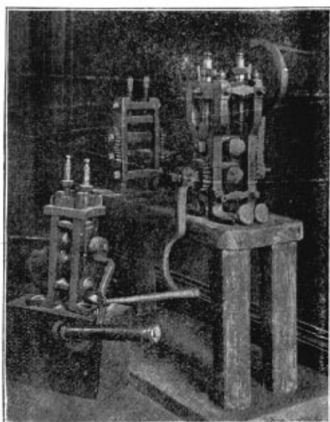
Stará »štreka«, Kapsové stroje (zadní z r. 1630, přední z r. 1658), z Eggenbergské mincovny na Krumlově.
