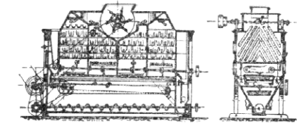
»Optima«, stroj na čištění krupic a krupiček.
