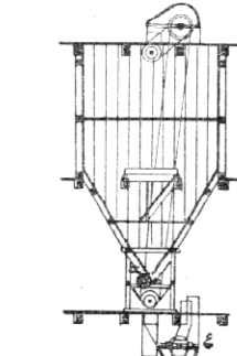
Stroj na mísení mouky.
