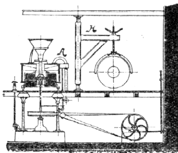
Mlýnské složení hnané řemenem.
