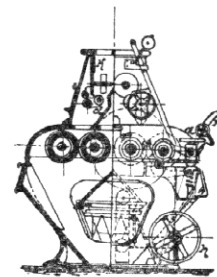
Stolice čtyřválcová.
