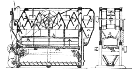
»Reforma«, stroj na čištění krupic a krupiček.
