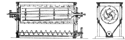
Vysejvač odstředivý.
