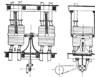
Dvojitý vysejvač rovinný.
