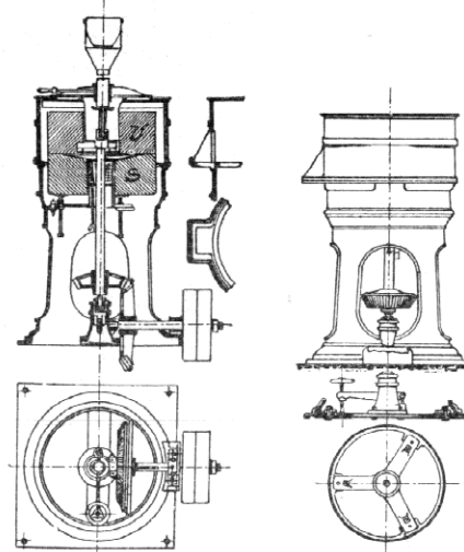
Mlýnské složení hnané soukolím.
