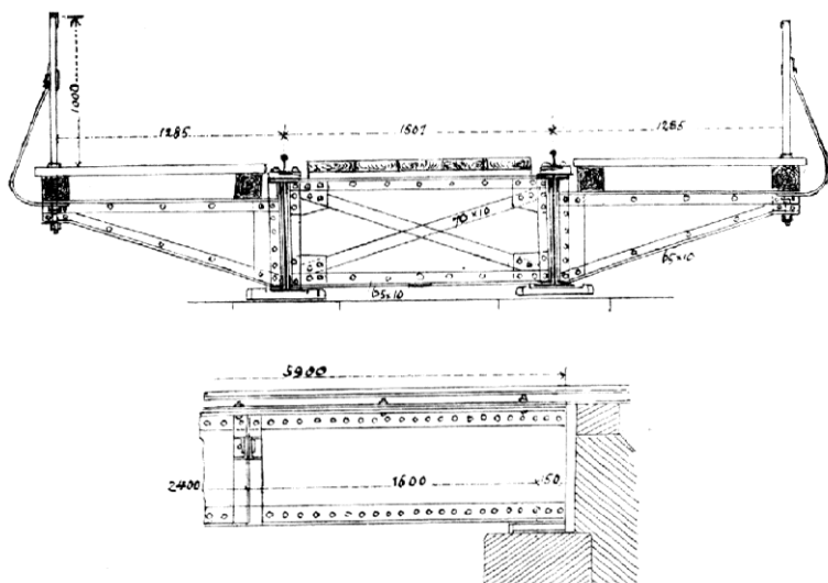
Plechový (trámový) most nad železniční propustkou, světlost 5.9 m.
