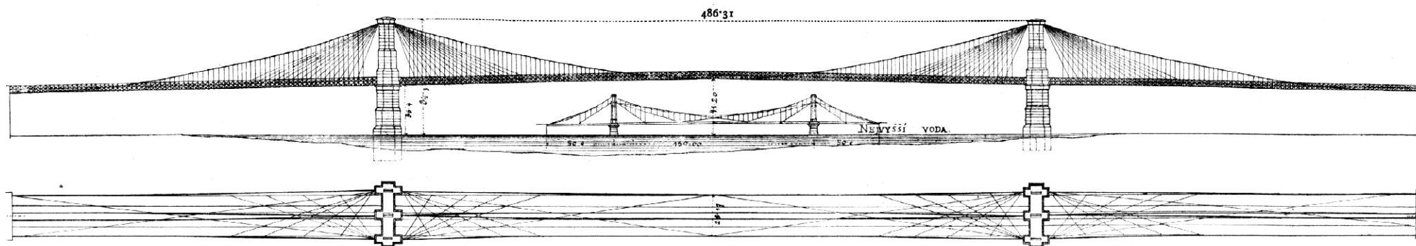
Visutý most přes East River mezi Brooklynem a New-Yorkem. Přirovnání s mostem císaře Františka Josefa v Praze. (Stejné měřítko od stejné hladiny vodní.)
