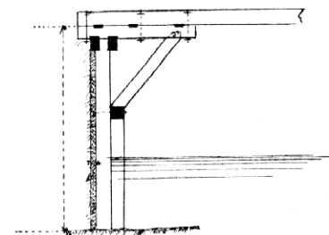
Dřevěná opěra pobřežní (do výše 5-6 m).
