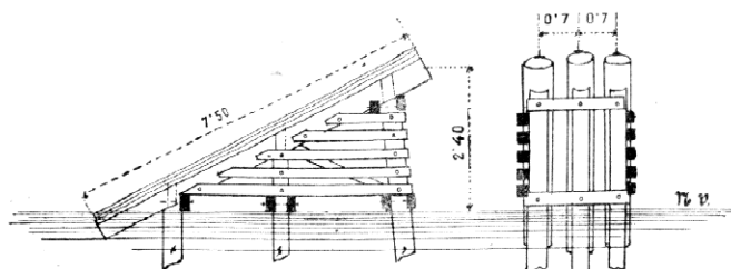
Ochranná koza, ledoborec (dle provedení při mostě u Národ. divadla v Praze).
