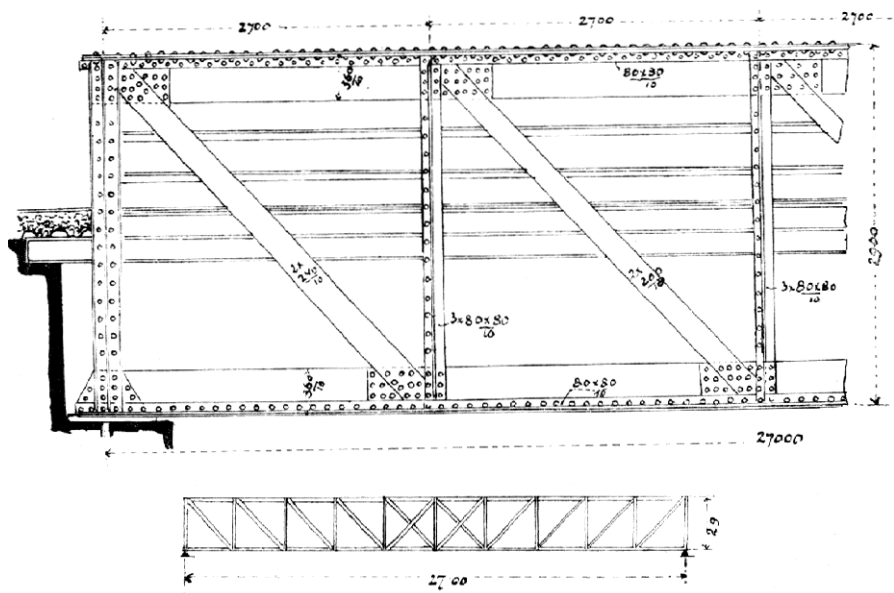
Pohled na část silničního železného mostu přes Sázavu v Koceradech (přímopásová soustava); světlost 27 m.
