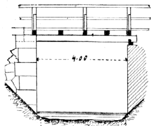
Dřevěná lávka (světlost 4 m).
