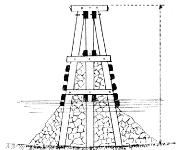
Dřevěná opěra návodní (do výše až 9 m).
