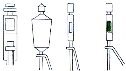
Výměna postavena na přímou, jede-li se po hrotu jede-li se proti hrotu .
