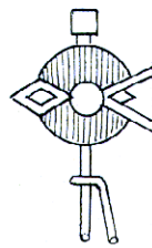
Výměna postavena do odbočky na levo, jede-li se proti hrotu .
