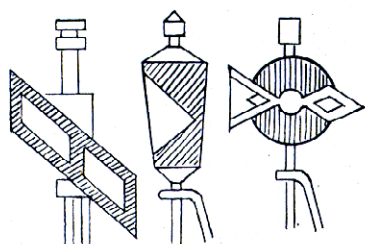
Výměna postavena do odbočky na pravo, jede-li se proti hrotu .
