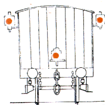
»Zadek« vlaku za tmy.
