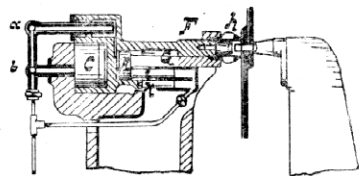
1. Řez válcem nýtovacího stroje Tweddellova.
