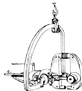
6. Přenosný nýtovací stroj Tweddellův.
