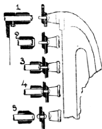
2. Postup práce na nýtovacím stroji Tweddellově.
