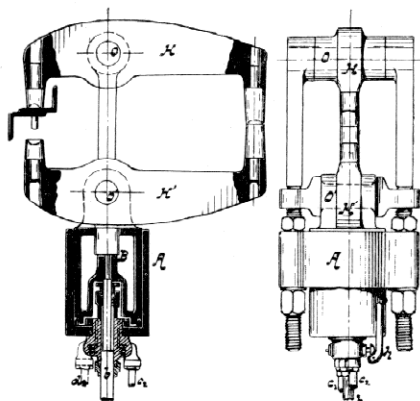
4. a 5. Přenosný nýtovací stroj Tweddellův.
