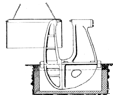
9. Nýtování nádržek strojem.
