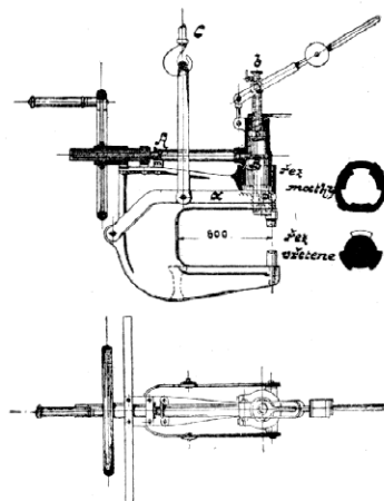
13. Delaloeuv nýtovací stroj ruční.
