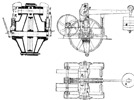
14., 15. a 16. Prášilův stroj nýtovací, poháněný transmissí.
