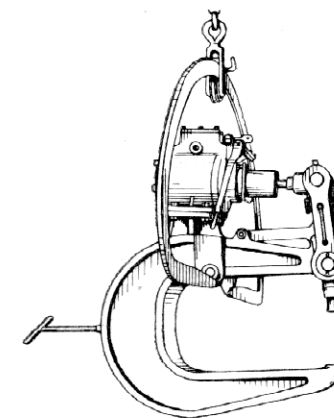
11. Nýtovací stroj pneumatický.
