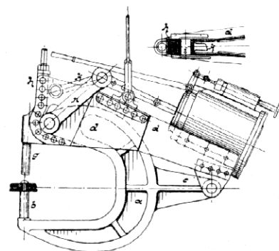
12. Nýtovací stroj pneumatický.
