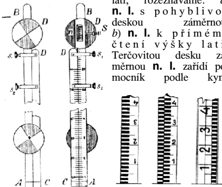
Č. 2886. Nivellační lat' s terčovitou deskou záměrnou.
