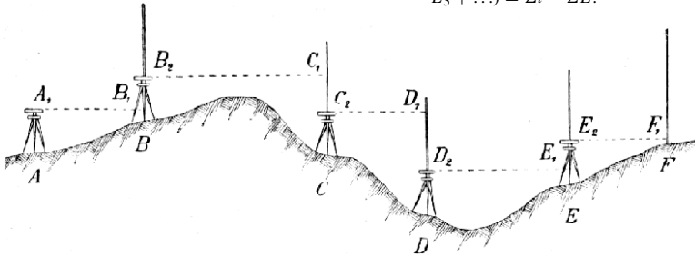
Č. 2899. Geometrická nivellace ku předu.
