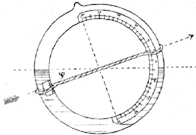
Č. 2895. Svahoměr prstencový.
