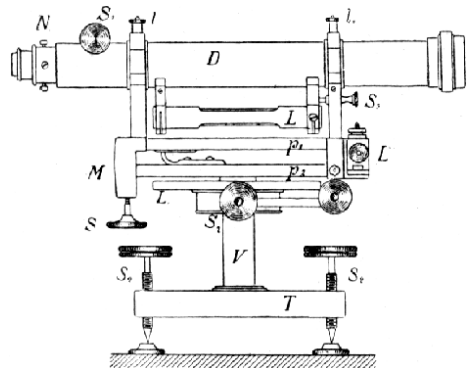
Č. 2897. Fricův nivellační stroj.
