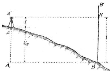
Č. 2898. Nivellace obyčejná.
