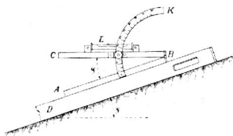
Č. 2890. Svahoměr obyčejný.
