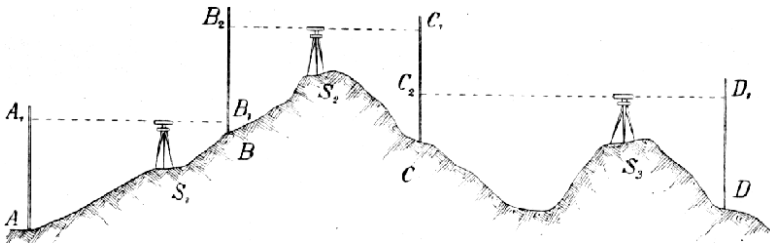
Č. 2900. Geometrická nivellace ze středu.
