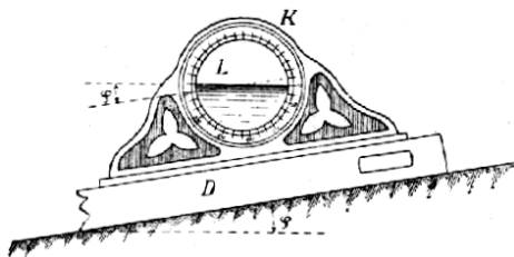
Č. 2892. Svahoměr americký.
