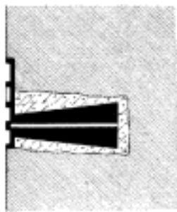
Č. 2902. Výšková značka řádu prvního.
