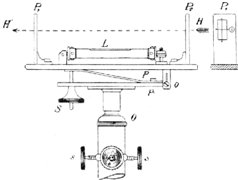
Č. 2896. Wegův nivellační dioptr.
