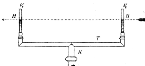
Č. 2893. Svahoměr trubcový (dvouramenný).
