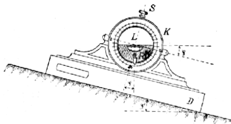
Č. 2891. Svahoměr Dawisův.
