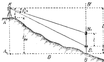
Č. 2901. Trigonometrická nivellace.
