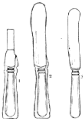
Č. 2906. Postup výroby nože při válcování.
