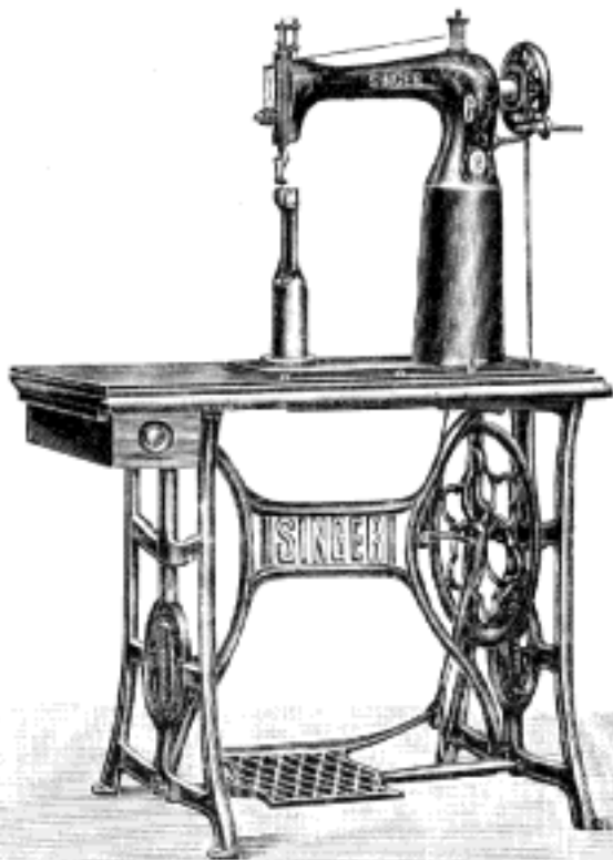
Č. 2937. Obuvnický stroj sloupkový.
