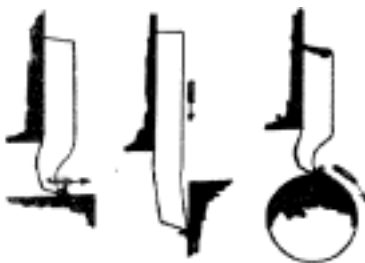
3 Č. 2913. Nože obráběcí. 1. při hoblování, 2. při obražení, 3. při soustruhování.
