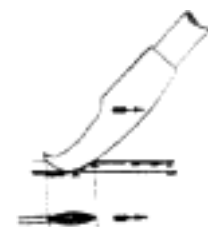
Č. 2909. Řezák truhlářský.
