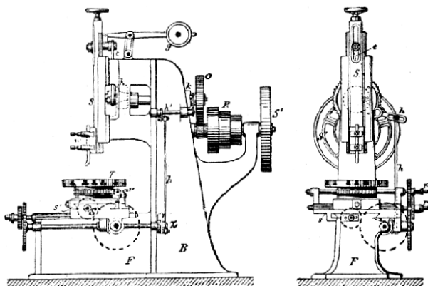
Č. 2935. Obrázecí stroje.
