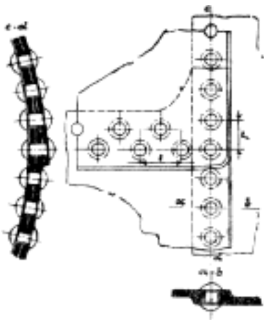
Č. 2931. Nýtové spojení plechů kotlových.
