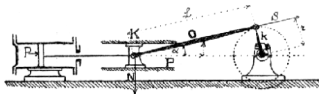
Č. 2948. Ojnice.
