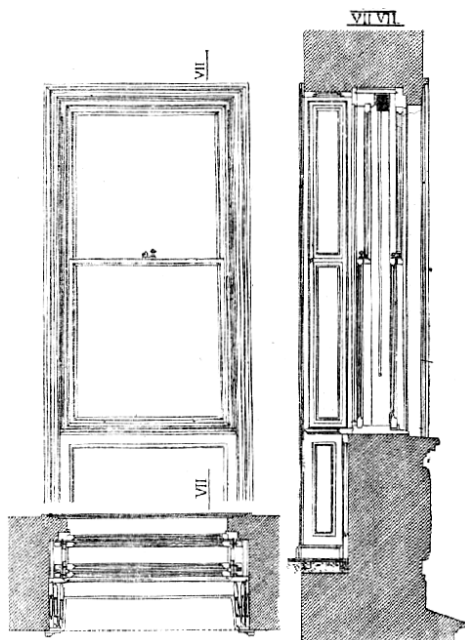
Č. 2953. Okno posouvací s vnitřní okéníci.
