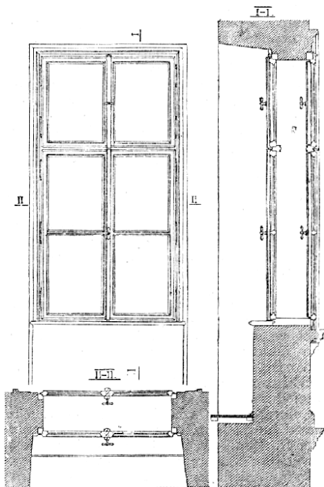
Č. 2951. Okno na venek se otevírající.
