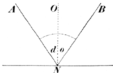
Č. 2943. Odraz světla.
