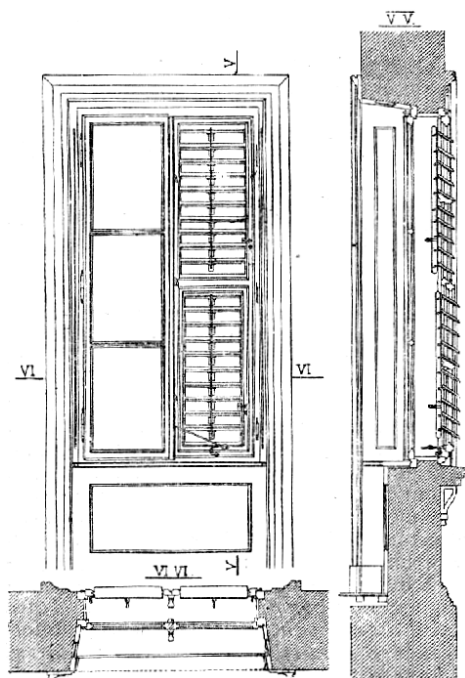
Č. 2950. Okno na venek se otevírající s jalousiemi.
