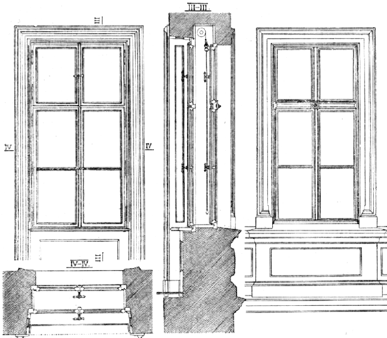
Č. 2952. Okno do vnitř se otvírající.
