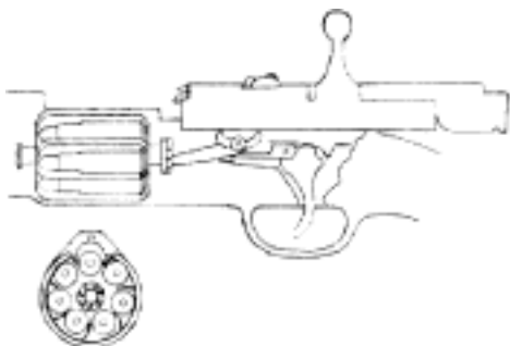
Č. 2960. Opakovačka Spitalského s průřezem válce.
