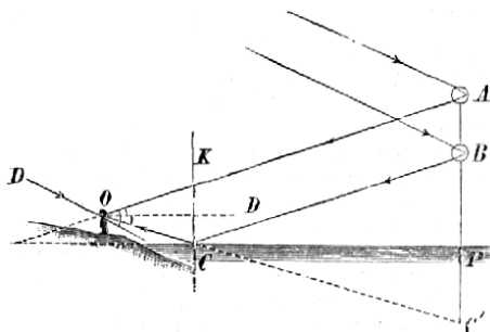
Č. 1250. Zrcadlení se duhy ve vodě.
