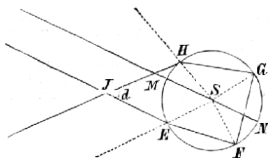
Č. 1249. Duha vedlejší.
