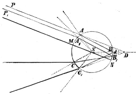
Č. 1248. Vznik duhy.
