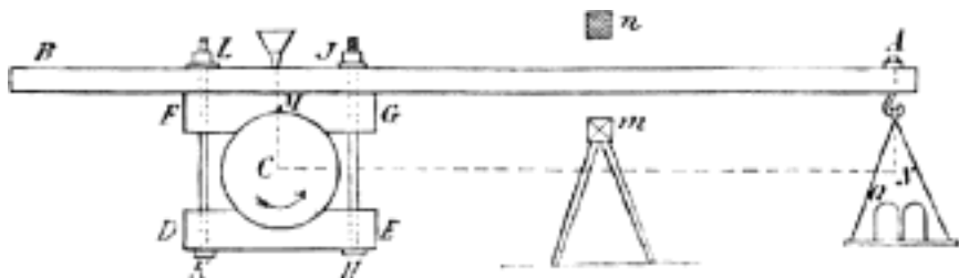
Č. 1278. Dynamometr Pronyho.
