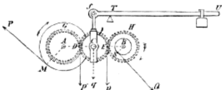
Č. 1276. Hachettovy dynamometrické vážky.
