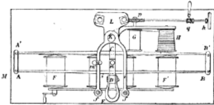
Č. 1274. Dynamometr Morinův.
