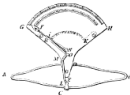
Č. 1273. Danamometr Regnierův.
