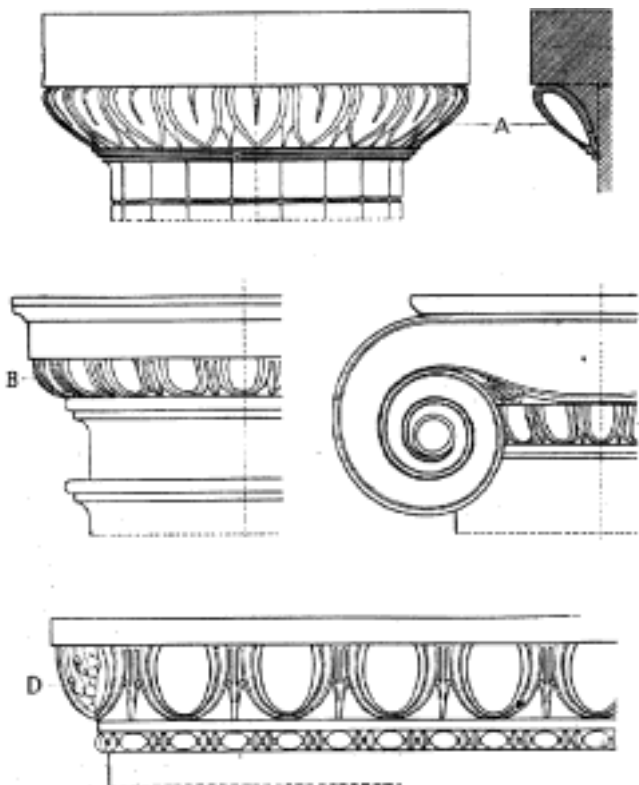
Kreslil řed. Dokoupil. Č. 1312. Echinus: A) ech. řecko-dórské hlavičky, zdobený polychromovaným listem; B) ech. římsko-dórské hlavičky, zdobený plastickým vaječníkem; C) ech. iónské hlavičky, zdobený plastickým vaječníkem; D) římsový člunek echinový, plasticky vaječníkem zdobený.
