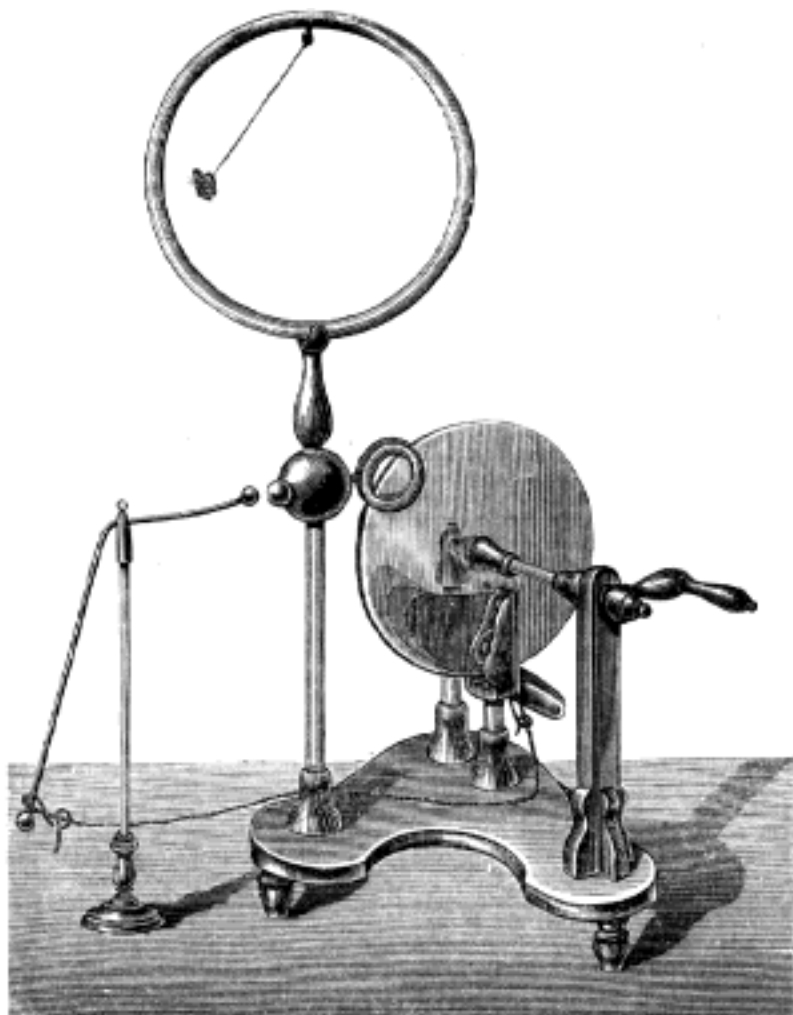
Č. 1334. Elektrika Winterova, dle provedení firmy Houdek v Praze.
