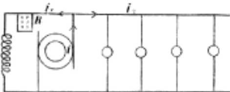
Č. 1328. Schema elektrického stroje derivačního.
