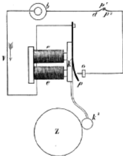
Č. 1332. Elektrické zvonítko.
