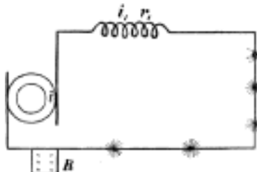
Č. 1327. Schema elektrického stroje seriového.
