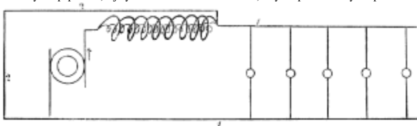
Č. 1329. Schema elektrického stroje compoudního.
