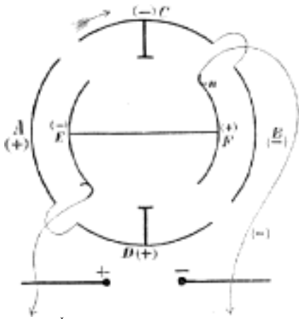
Č. 1333. Schema elektriky influenci.
