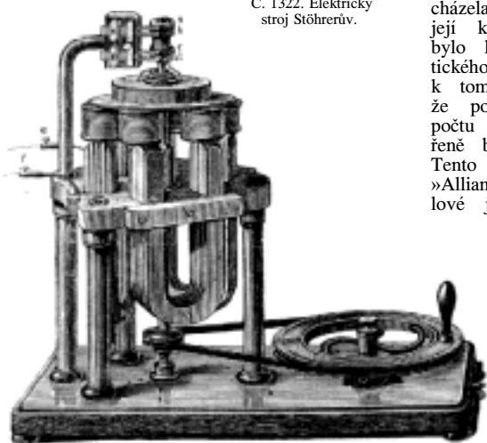
Č. 1322. Elektrický stroj Stöhrerův.
