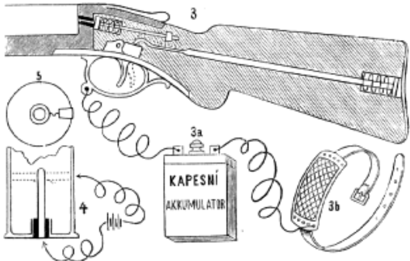
Č. 1331. 3. Elektrická ručnice Pieperova s kapesním akumulátorem (3a) a síťkou (3b). - 4. Průřez nábojnice téže. - 5. Zátka k nábojnici.
