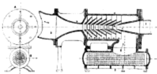
Č. 1316. Ejektor Friedmanův.
