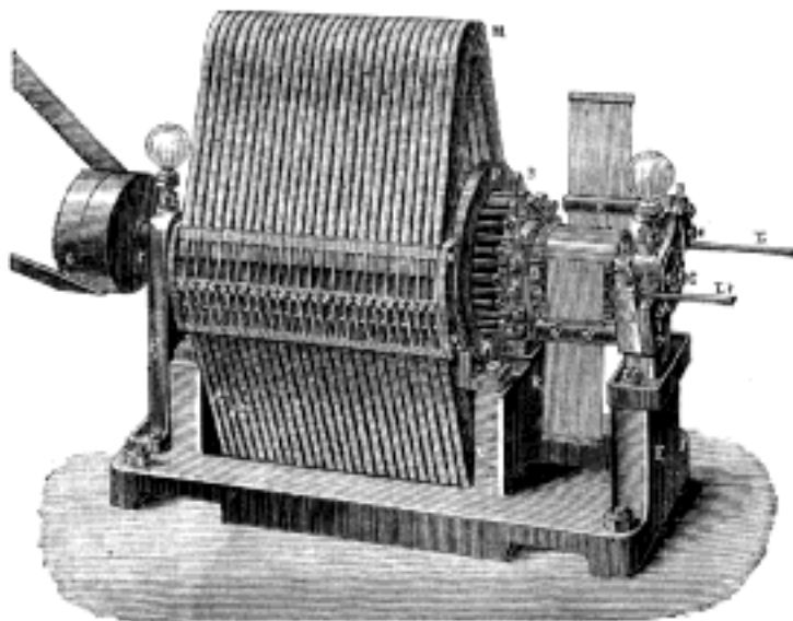
Č. 1325. Magneto elektrický stroj Siemensův.
