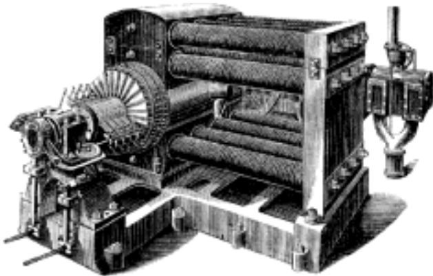
Č. 1326. Edisonův stroj dynamoelektrický.
