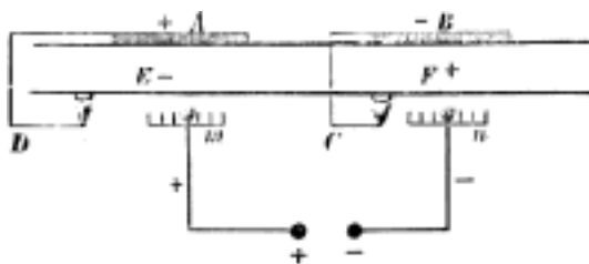
Č. 1336. Schema elektriky Toeplerovy.
