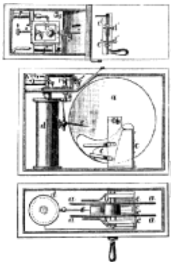
Č. 1338. Polní elektrický stroj zapalovací.
