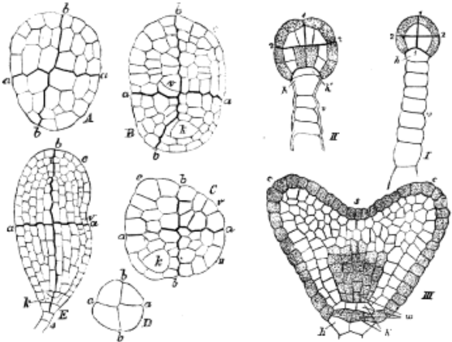
Č. 1350. Embryo. A) Embryo tobolky jatrovkovitého mechu Marchantia , rozdělený dvěma prvními příhradkami aa, bb ve 4 kvadranty. B) Embryo kapradiny Ceratopteris : 2 hoření kvadranty dají dělohu c; v první buňka stonku, k konečná buňka kořene. C) Embryo kapradiny Pteris : c, v, k jako přvé, n noha. D) Týž embryo v prvo počátku, čtyřbuněčný. E) Embryo jednoděložné rostliny Alisma : děloha c ze dvou hoření kvadrantů konečná, v vegetační bod stonku, k počátek kořenu, s suspensor. Embryo dvouděložný kokosky ( Capsella ), I, II., III. po sobě jdoucí stadia vývoje; v suspensor; h hypophysa, t. j. buňka přechodní mezi embryem a suspensorem; h její hoření, čepičku kořenu dávající segment; w kořen; cc obě dělohy; s úhel, v němž vzniká vegetační bod stonku; 1-1, 2-2 první dvě příhradky mezi čtyřmi kvadranty. Dermatogen (mladá pokožka) a plerom (pletivo vnitřní, z něhož svazky cévní se tvoří) jsou vystíněny.
