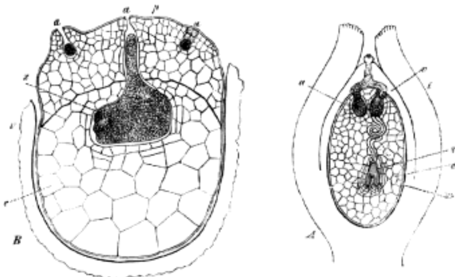
Č. 1354. Endosperm. B) Mikrospora Selaginelly: v protřezané vnější blána výtrusu (exosporium); p prothallium; a jeho archegonie; z zárodek (embryo), vyvinuvší se z centrální buňky prostředního archegonia, na suspensoru zavěšený a do endospermu e vrostlý. A) Vajíčko (zárodek semena) Conifery v podélném řezu: i integument; v jádro vaječné čili velkovýtrusnice; m makrospora čili vak klíční; e endosperm vyplňující makrosporu; a archegonie čili corpuscula, zúrodněné pylovým vakem, jenž vyrostl z pylového zrnka, na vrcholku jádra spočívajícího; z jednoho archegonia vzniknul zárodek neb embryo z na točitém suspensoru zavěšený.
