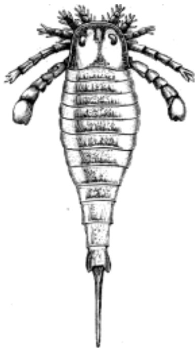
Č. 1394. Eurypterus Fischeri Eichw., ze svrchního siluru na ostrově Ezelu, zmenš.
