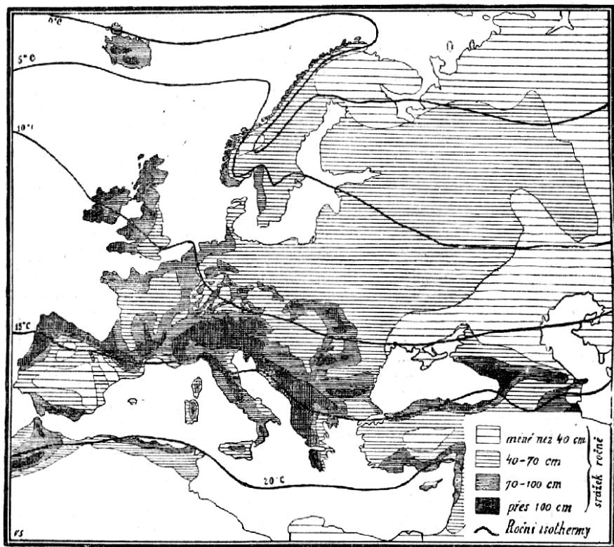
Č. 1398. Déšť a roční isothermy v Evropě.
