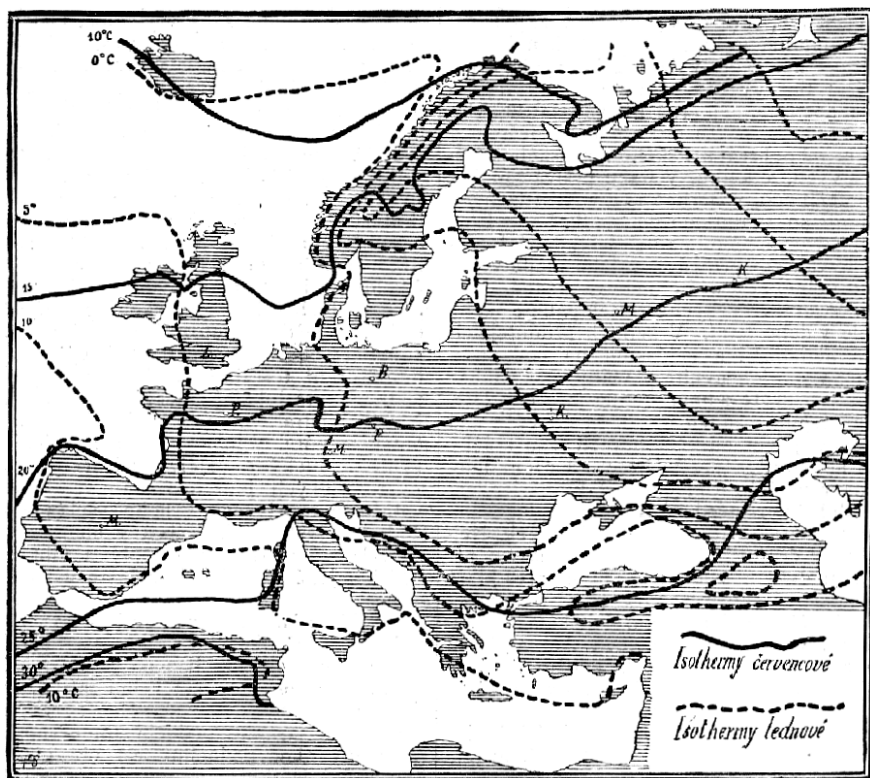
Č. 1399. Červencové a lednové isothermy v Evropě.
