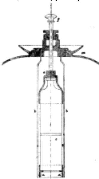
Č. 1415. Extincteur Dickův.
