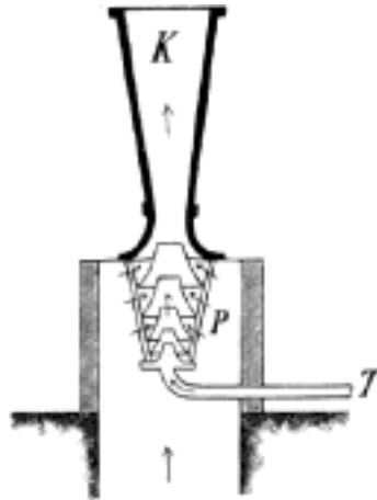
Č. 1410. Exhaustor Körtिंगův.
