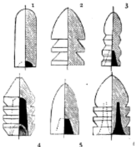
Č. 1412. 1) Moderní střela s »odtěžující dutinou«. 2) Kompressivní střela dle Charrina. 3) Expansivní střela dle Buholzera. 4) Expansivní střela s klínkem dle Minié. 5) Expansivní střela bez klínku dle Pritcheta. 6) Expansivní střela bez klínku dle Pritcheta.
