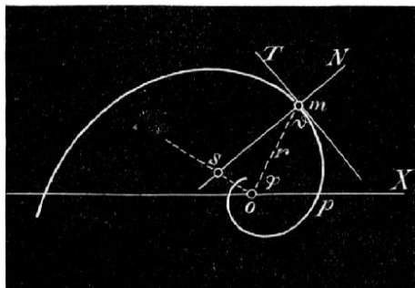
Č. 1414. Exponenciální spirála.
