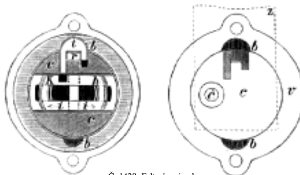
Č. 1428. Felterův zámek.
