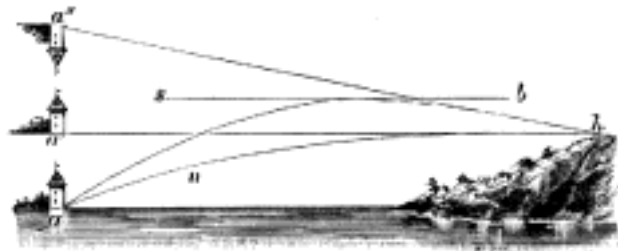
Č. 1426. Zrcadlení horní.
