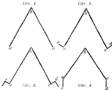
Č. 1442. Flèche v půdorysu. Obr. 1. Flèche prosté. - Obr. 2. Flèche s boky ku předu zahnutými. - Obr. 3. Flèche s boky lomenými. - Obr. 4. Flèche s boky na zad zapřenými. - ab, bc líce; ea, ed boky čili flanky; b, b, b, b hrot.
