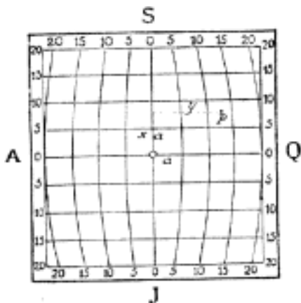
Č. 1441. Flamsteedova projekce.
