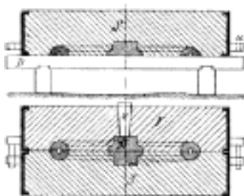
Č. 1453. Formování v rámu.
