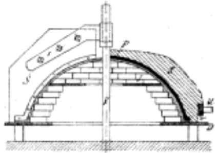
Č. 1455. Formování šablonou.
