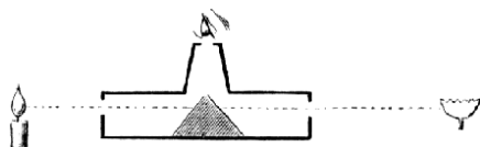
Č. 1461. Ritchieův fotometr.
