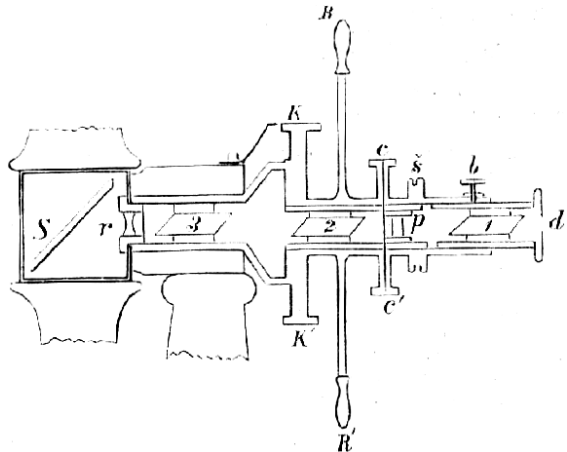
Č. 1465. Přístroj polarisáční.
