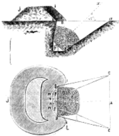
Č. 1469. Fougasse.
