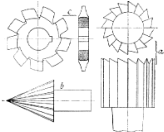
Č. 1482. Frésy na kovy.
