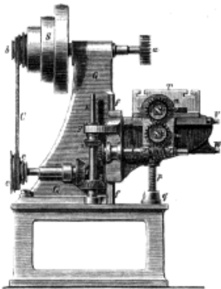
Č. 1484. Frésovací stroj na kovy.
