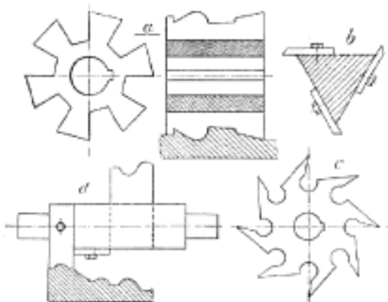
Č. 1483. Frézy na dřevo.
