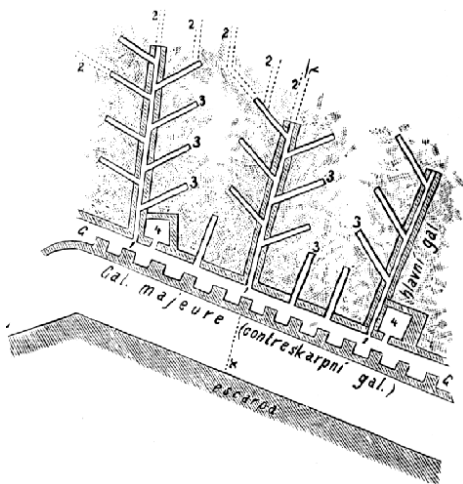
Č. 1504. a) Galerie ve hradebnictví.
