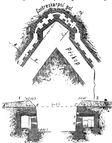
Č. 1503. Galerie ve hradebnictví.
