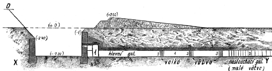
Č. 1504. b) Galerie ve hradbnictví.
