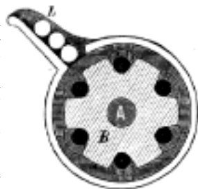
Č. 1534. Gatlingův kulomet: příčný řez s válcem nabíjecím.
