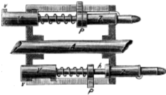
Č. 1535. Gatlingův kulomet: zařízení zámek.
