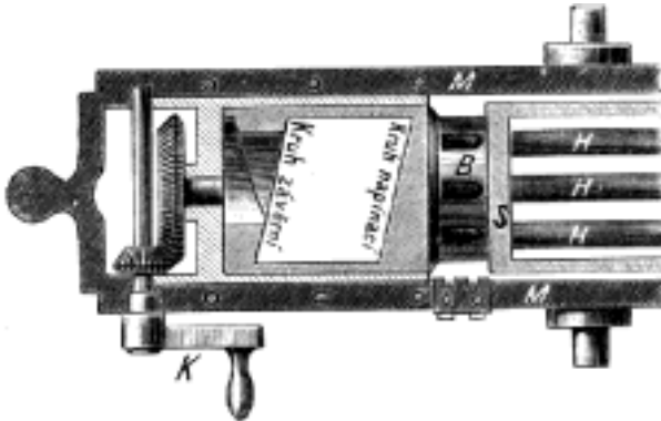
Č. 1536. Gatlingův kulomet: pohled shora, s částečným průřezem.
