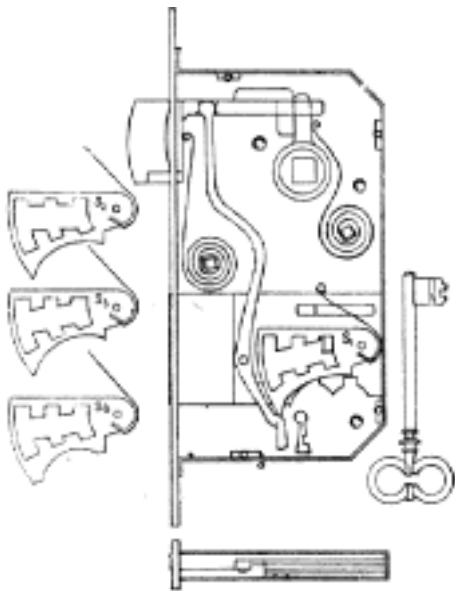
Č. 1529. Zámek chubb'ský s garniturou.
