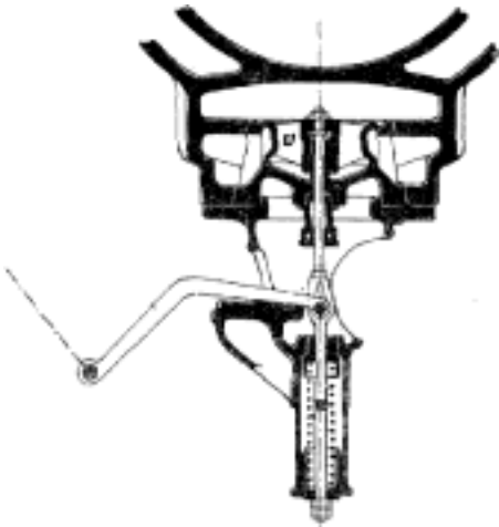
Č. 3591. Vypouštěcí ventil od rozvodu ventilového.
