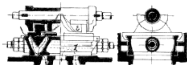
Č. 3588. Rozvod Guhrauerův.
