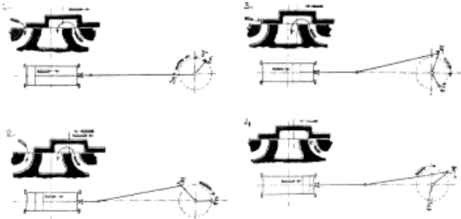
1. Pist v krajní poloze v levo, levý kanál vpuštěcí otevřen o lineární předstih vpuštěcí, pravý kanál o lineární předstih vypouštěcí.
