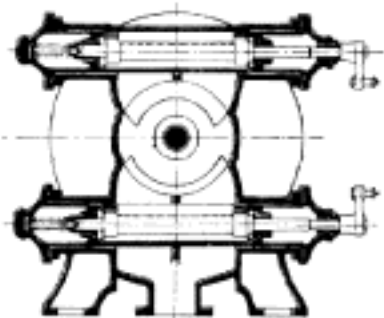
Č. 3593. Uspořádání vřetovitých šoupátek při rozvodu Corlissově.
