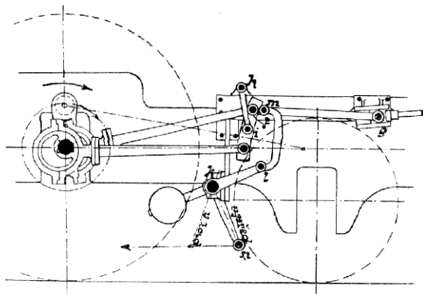
Č. 3595. Vratný rozvod Stephensonův. Č. 3596. Vratný rozvod s kulisou Goochovou.
