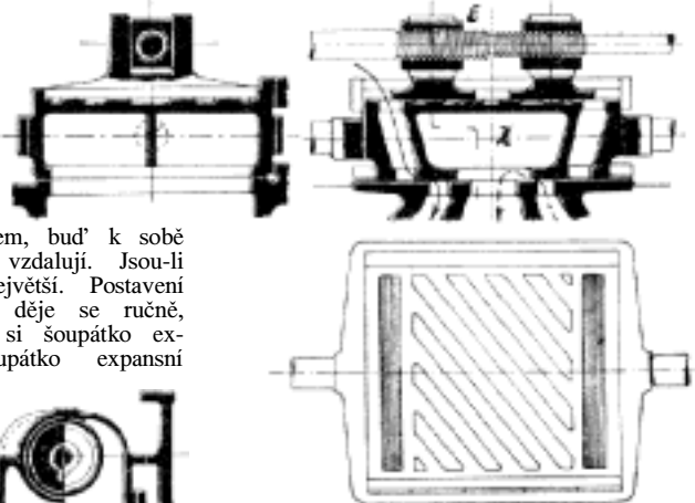
Č. 3585. Rozvod Meyerův.
