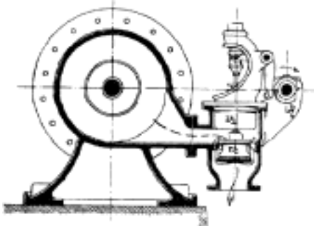
Č. 3592. Rozvod ventilový s neokrouhlými kotouči.
