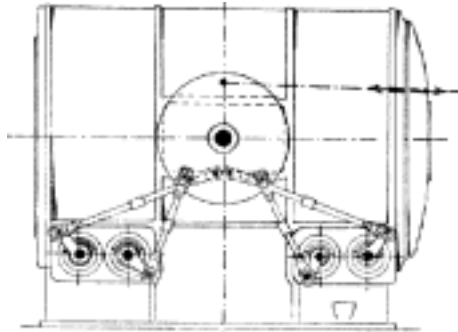
Č. 3594. Rozvod Corlissův s kohouty na zpodku válce.
