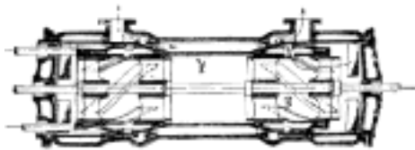
Č. 3590. Rozvod Riderův. Obě šoupátka pístová.
