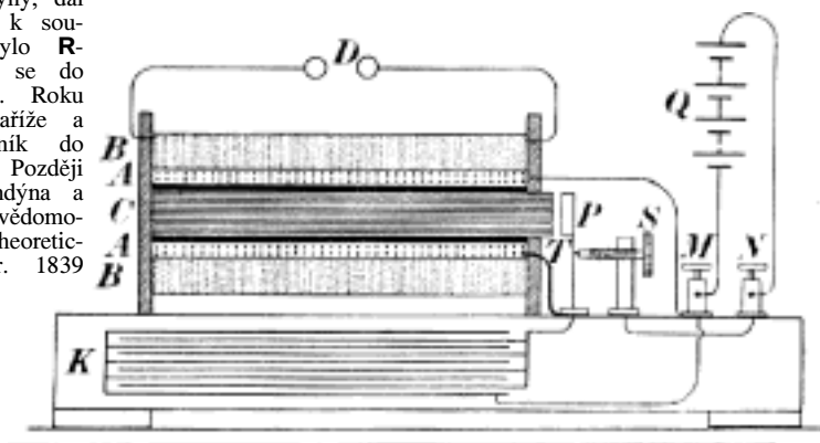
Č. 3605. Ruhmkorffův induktor.
