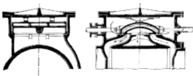
Č. 3589. Šoupátka Trickova.
