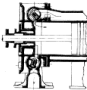
Č. 3593. Uspořádání vřetovitých šoupátek při rozvodu Corlissově.
