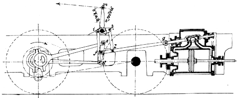
Č. 3597. Vratný rozvod s kulisou Allanovou.
