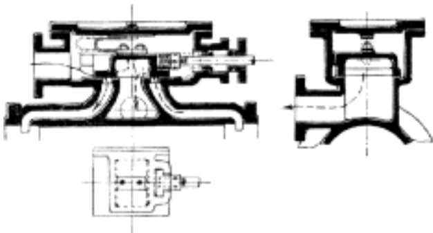
Č. 3583. Řez šoupátkovou komorou se šoupátkem jednoduchým.
