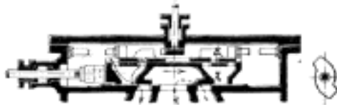
Č. 3587. Rozvod Farcotův.
