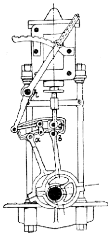
Č. 3595. Vratný rozvod Stephensonův. Č. 3596. Vratný rozvod s kulisou Goochovou.
