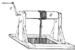
Č. 3610. Rumpál.
