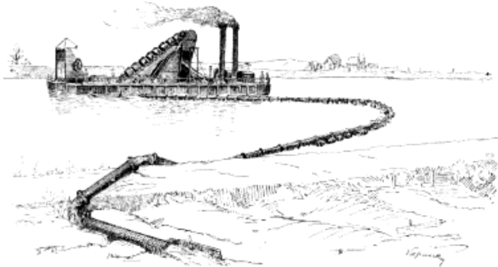
Č. 3642. Skládání potrubím plovoucím.
