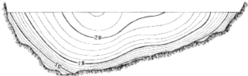
Č. 3635. Měření rychlosti v Labi u Děčína při stavu vody +1.321 m vodočtu děčínského.
