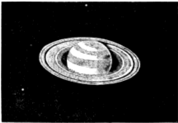
Č. 3682. Saturn.
