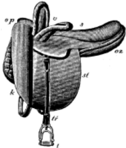
Č. 3701. Sedlo dámské: k kolenice; op oblouk přední; oz oblouk zadní; s sedadlo; st stranice; t třmen; tf třmenice; v vidlice.
