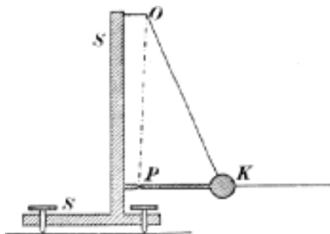
Č. 3705. Seismometr.
