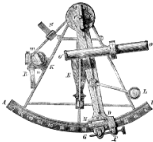
Č. 3718. Sextant zrcadlový.
