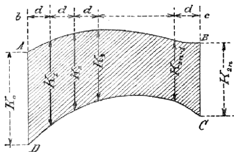
Č. 3738. Simpsonovo pravidlo.
