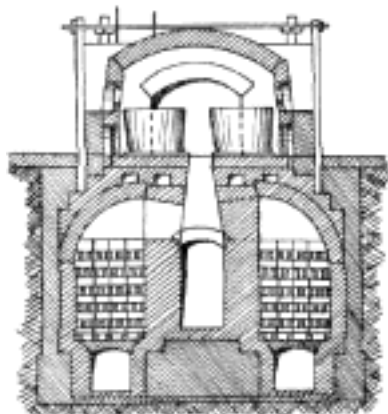
Č. 3765. Siemensova sklářská pec regenerátorová. Řez příční.
