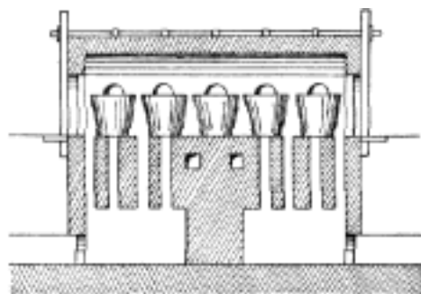
Č. 3766. Siemensova sklářská pec regenerátorová. Řez podélný.
