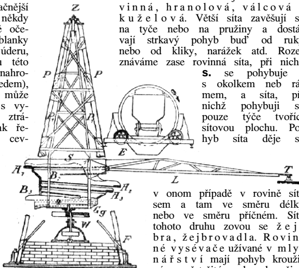
Č. 3750. Sdružovací síto Karlíkovo.
