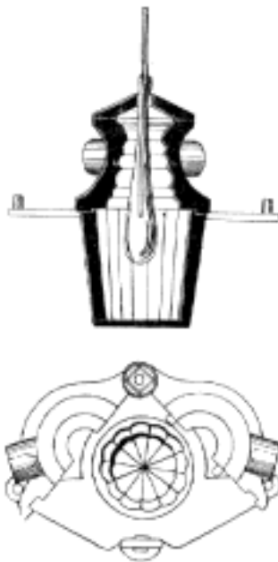
Č. 3770. Forma na láhev.
