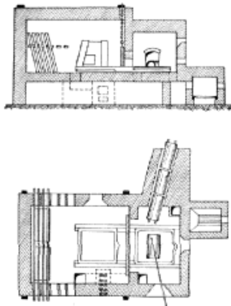
Řez podélný. Půdorys. Č. 3775. Pec narovnávací a chladicí.
