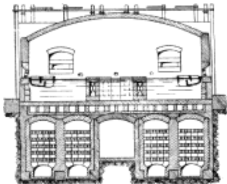
Č. 3767. Siemensova sklářská pec dvojvanová. Rez podélný.
