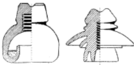
Č. 3746. Isolátor olejový. Č. 3747. Isolátor »Delta«.
