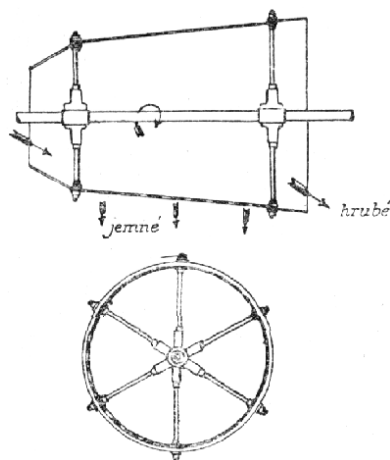
Č. 3752. Sítový buben kuželový.
