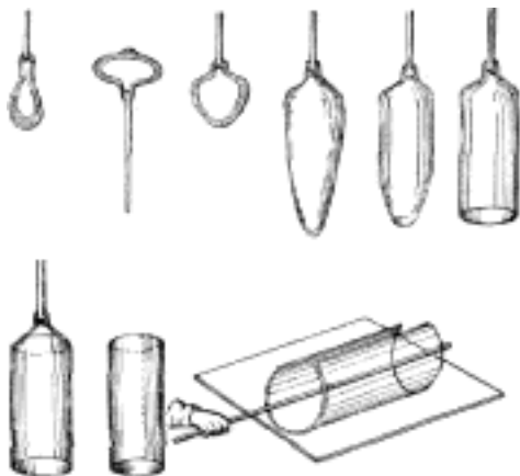
Č. 3774. Postup výroby foukaného skla tabulového.
