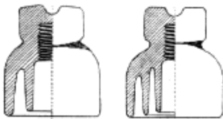
Č. 3744. Isolátor dvojplášťový. Č. 3745. Isolátor tříplášťový.
