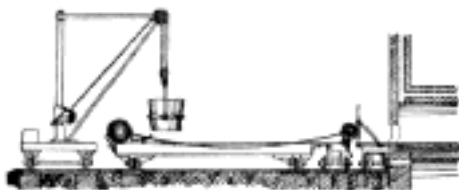
Č. 3776. Zařízení pro lití skla tabulového.
