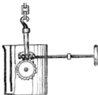
Č. 3791. Pánev jeřábová.
