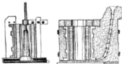
Č. 3795. Zaformování válce.
