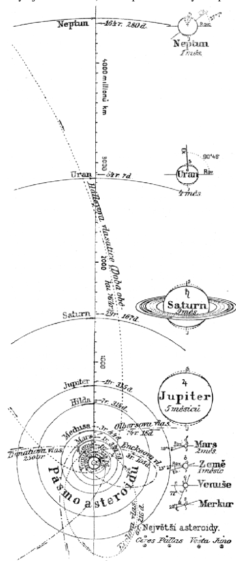
Č. 3807. Sluneční soustava.
