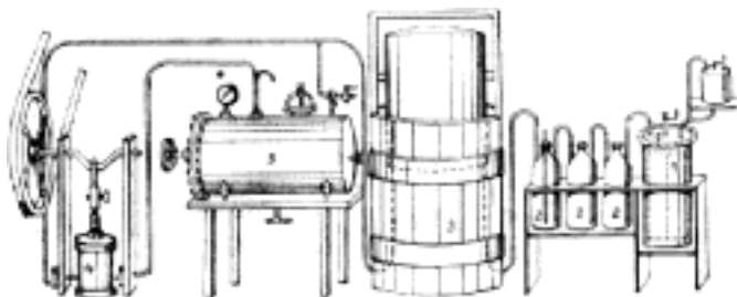
Č. 3822. Přístroj pumpový.
