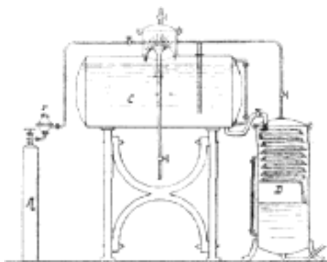
Č. 3824. Přístroj sodovkový s použitím tekuté kyseliny uhličitě.
