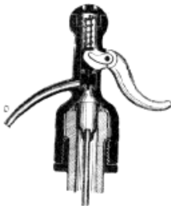
Č. 3821. Závěr sifonový.
