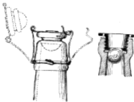
Č. 3819. Závěr příklopový. Č. 3820. Závěr kuličkový.
