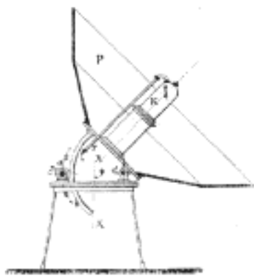
Č. 3825. Solární motor Pifréuv.
