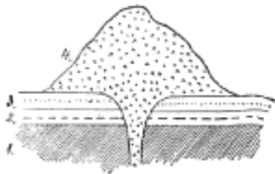
Č. 3834. Schematický průřez Ostrého u Milešova v Čechách. (Podle J. N. Woldřicha.)
