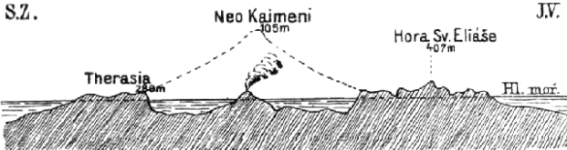
Č. 3836. Průřez Santorinem. Starý tvar sopky doplněn čárkami.
