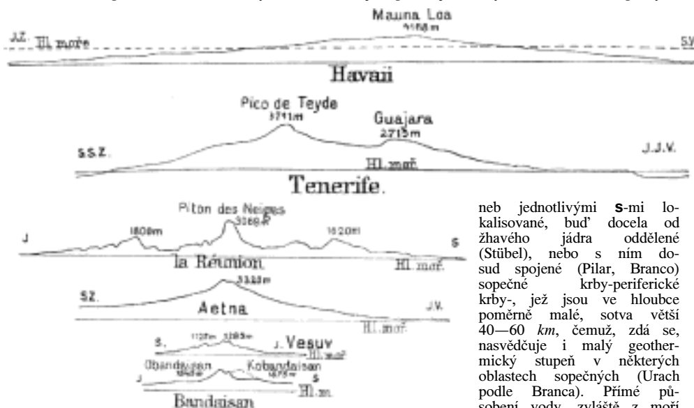
Č. 3837. Profily sopek v též měřítku výškovém a délkovém. Havaii 1:2,500,000, ostatní 1:500,000. Podle A. Pencka.
