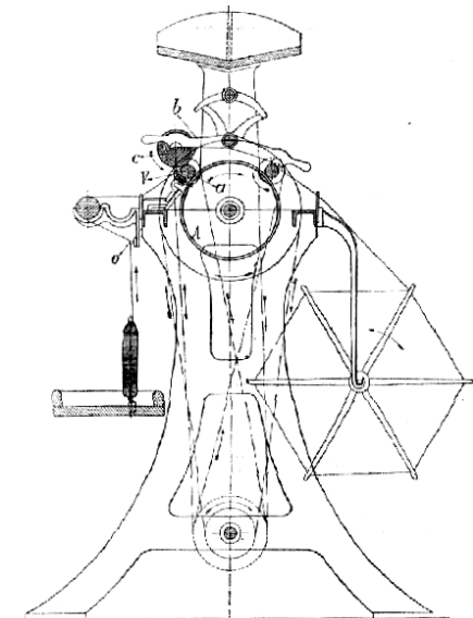
Č. 3848. Stroj křížem soukací.
