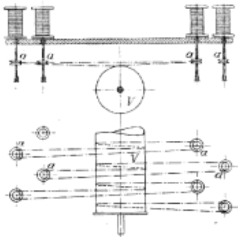
Č. 3846. Pohon stojatých vřeten soukacího stroje.
