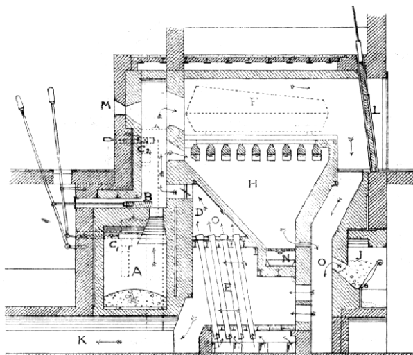
Č. 3868. Pec na spalování mrtvol v Offenbachu n. m. (soust. Klingenstierna-Beck).
