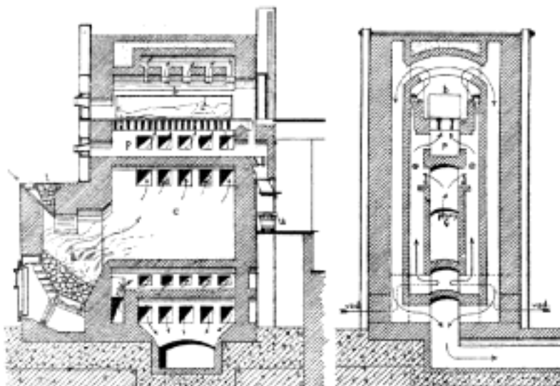
Č. 3867. Anglická pec na spalování mrtvol (sestr. Simon a Bourry).
