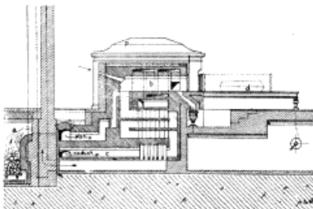
Č. 3864. Pec na spalování mrtvol v Curichu (setr. inž. C. E. Bourry).
