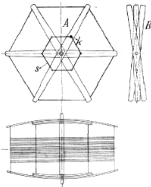
Č. 3842. Sklopný víjak s nasazeným přádenem; A rozložený a pojištěný šňůrou a s kolíkem k , B sklopený.
