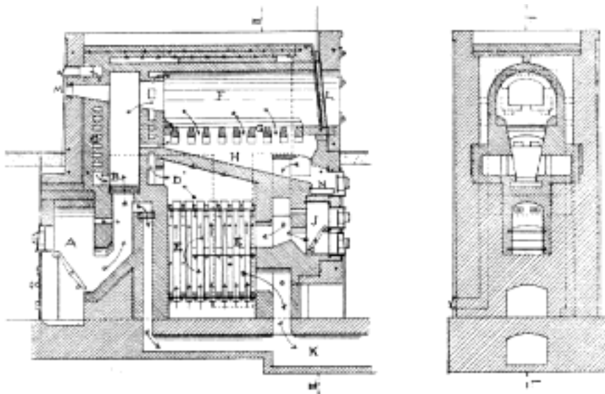
Č. 3869. Pec na spalování mrtvol v Mohuči (soust. Klingenstierna-Dorovius).
