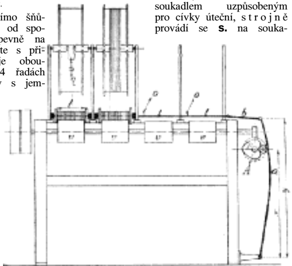
Č. 3844. Soukací stroj osnovný s cívkami ležatými.
