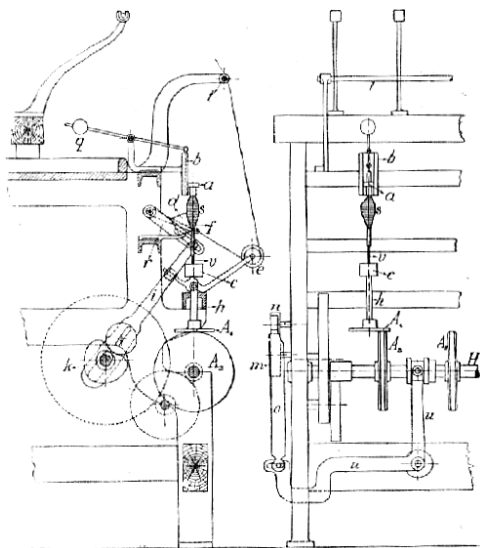
Č. 3849. Stroj soukací na útek.
