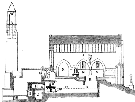
Č. 3870. Podélný řez krematoria v Glasgově.
