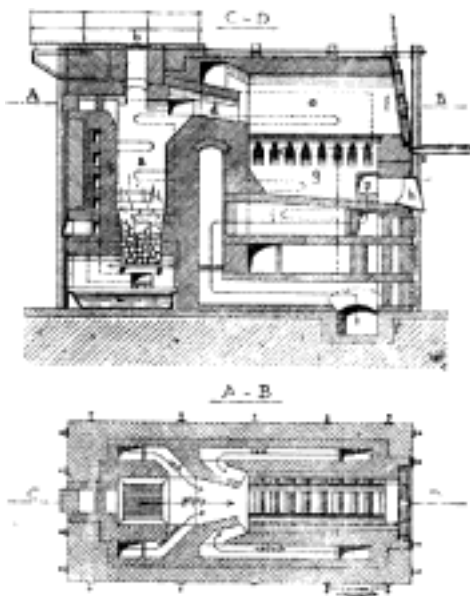
Č. 3865. Pec na spalování mrtvol (sestr. inž. Rich. Schneider).
