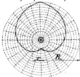
Č. 3845. Konstrukce neokrouhlého kotouče pro pohon vodiče.
