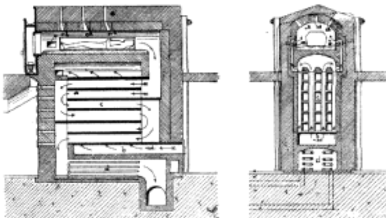
Č. 3866. Pec na spalování mrtvol svítíplynem (sestr. inž. Guichard).
