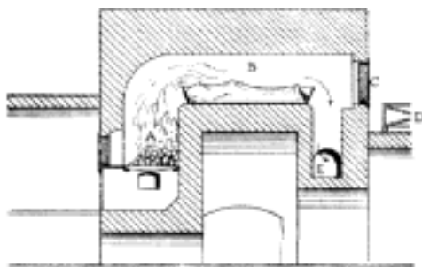
Č. 3860. Pec na spalování mrtvol podle prof. Goriniho.
