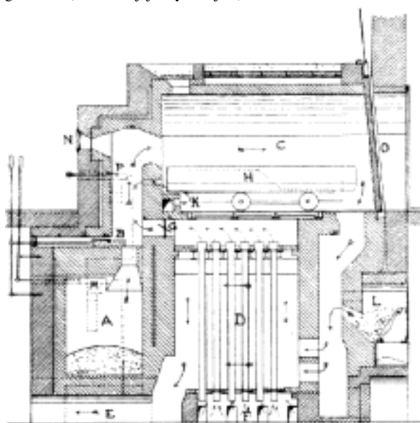
Č. 3863. Pec na spalování mrtvol v heidelbergce (sestrojil švéd. plukovník Klingenstierna).
