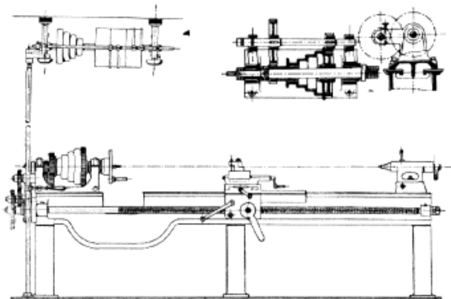
Č. 3855. Soustruh s vřetenem šroubovým. Č. 3856. Vřeteník.
