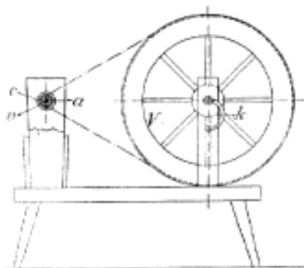
Č. 3841. Ruční soukadlo; v vřeten, c cívka, V hnací kolo, k klika poháněcí, a přeslen.
