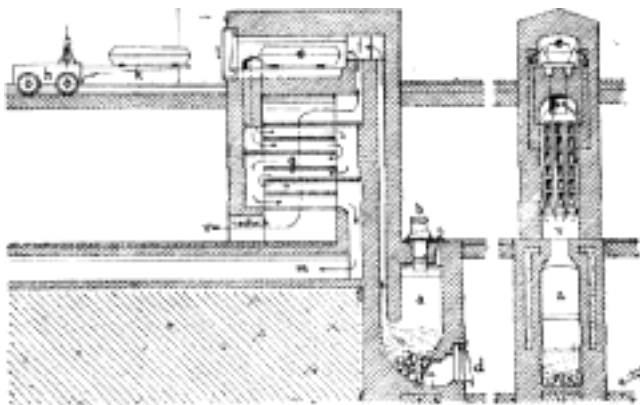
Č. 3862. Pec na spalování mrtvol v Paříži (sestrojil Toisoul a Fradet).
