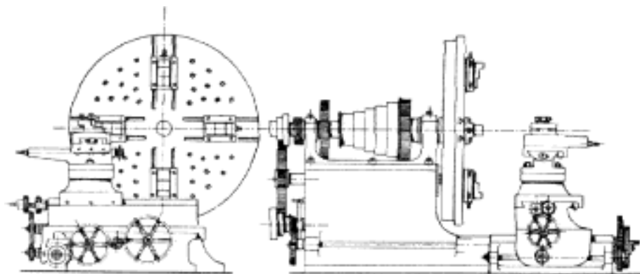
Č. 3858. Soustruh kusý.
