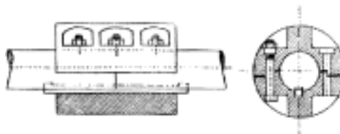
Č. 3891. Spojka misková.
