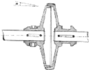
Č. 3896. Třecí spojka konická.
