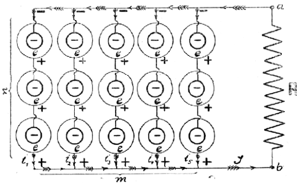
Č. 3886. Spojení smíšené.
