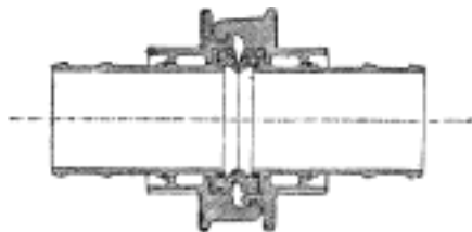
Č. 3904. Průřez spojky Knaustovy.
