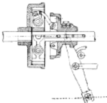
Č. 3897. Třecí spojka cylindrická.
