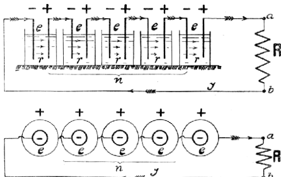
Č. 3884. Spojení za sebou.
