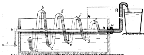
Č. 3882. Spirální pumpa.
