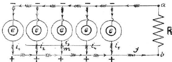
Č. 3885. Spojení vedle sebe.
