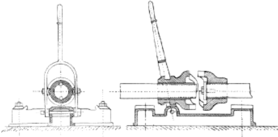
Č. 3895. Výsuvná spojka zubová.
