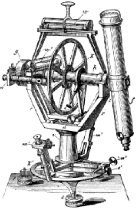
Č. 175. Altazimut
