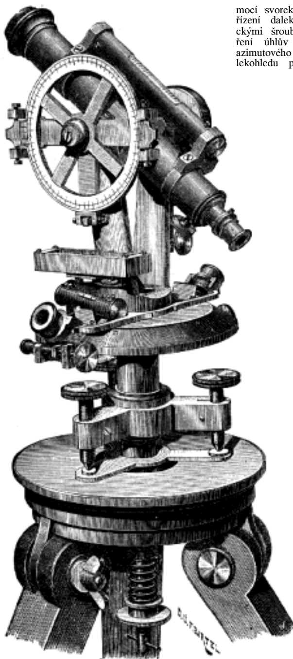
Č. 176. Altazimut
