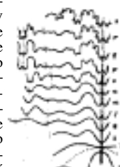
Č. 224. Švy ammonoidel pokračující starším ve složitosti (od g k s).
