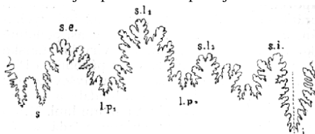
Č. 219. Čára švu ammonoidei. s. lok sifonální čili vnější nebo břišní, lp1, lp2 laloky postranní, i. lalok vnitřní, antisifonální nebo hřbetní, s.e. sedlo vnější, sl1, sl2 postranní sedla, s. i. sedlo vnitřní
